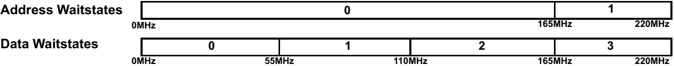
图 4-1. 等待状态机制
