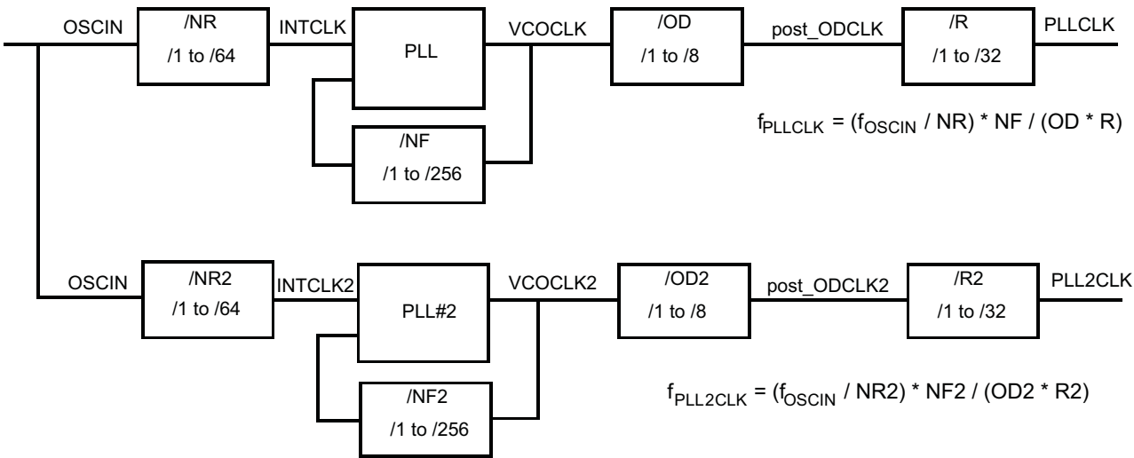
图 5-6. PLLx 方框图
