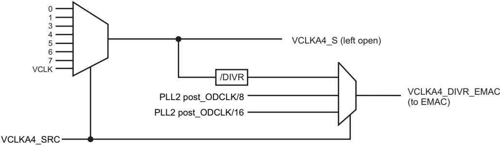
图 5-8. VLCKA4_DIVR 源选择选项
