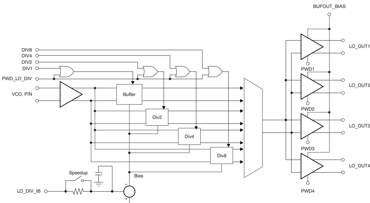
Figure 68. LO Divider
