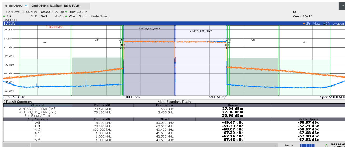
图 4. 情况 3：启用 DPD 之前（橙色）和之后（蓝色）的 ACLR 图
