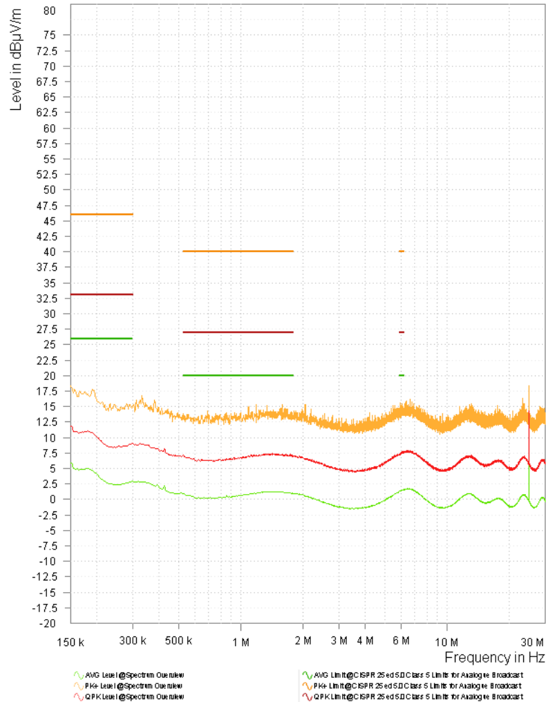
图 3-9. 型号 3 LMK3H0102-Q1 1.8V 频谱概述 - 单极
