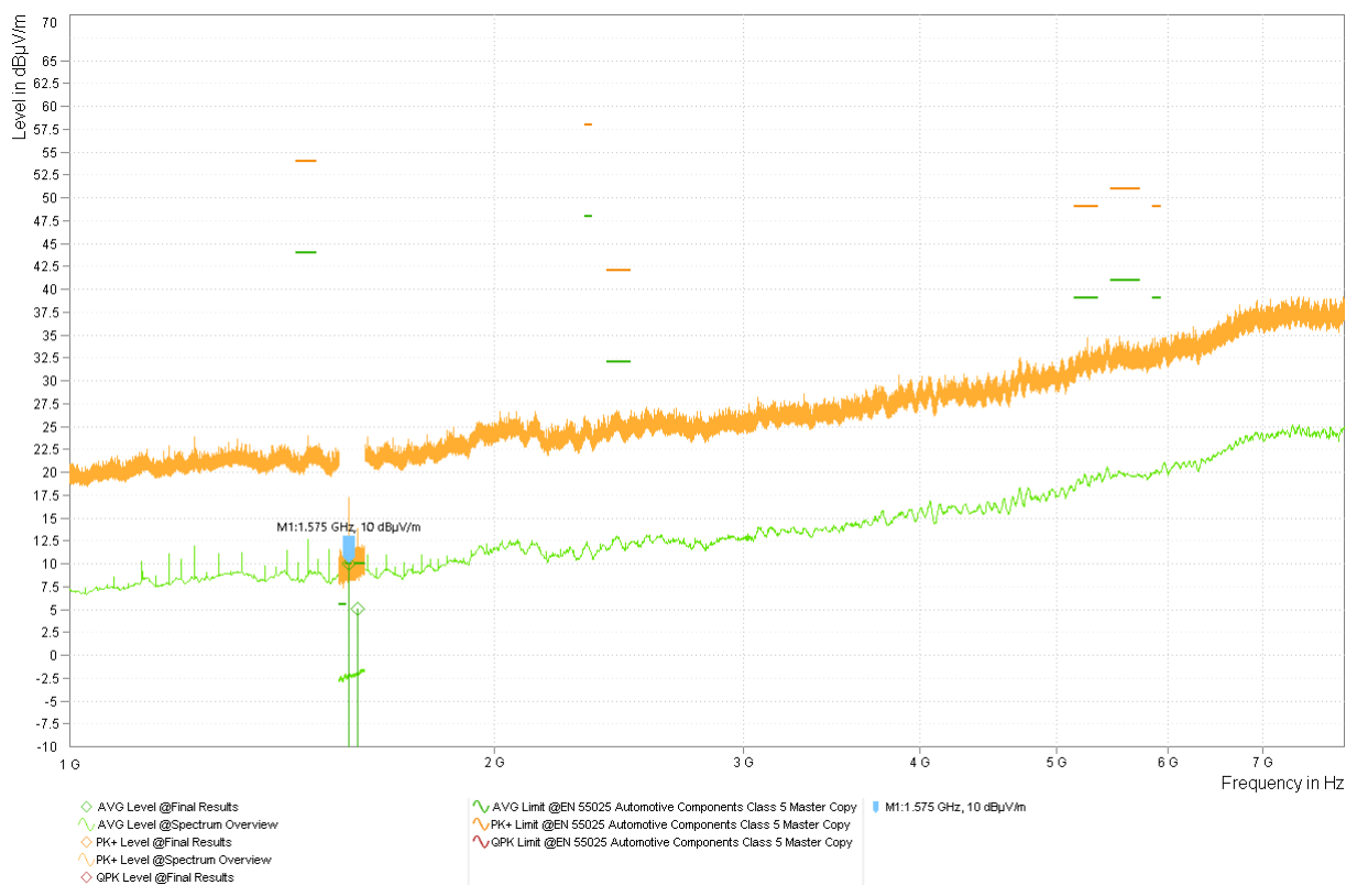
图 3-27. 型号 4 竞品振荡器 1.8V 频谱概述 - 喇叭
