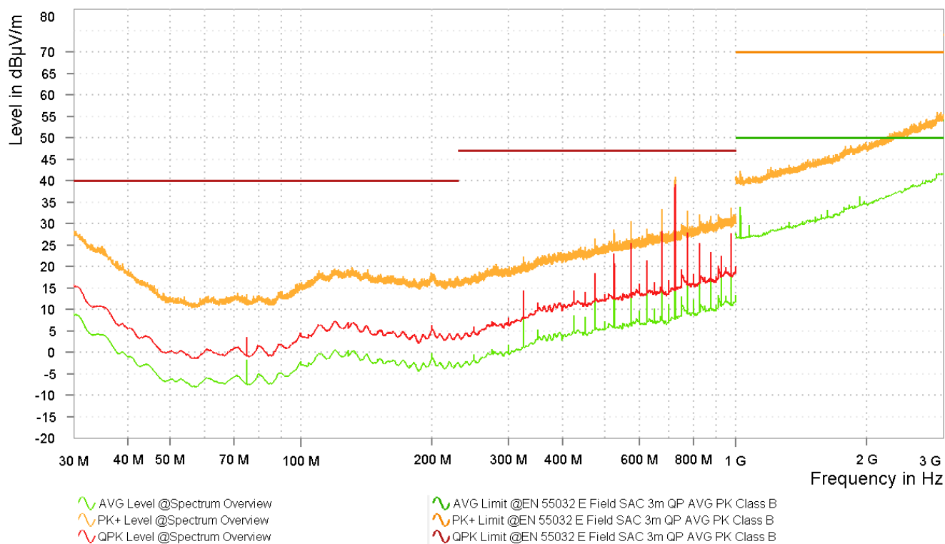
图 4-9. 型号 3 LMK3H0102-Q1 3.3V Z 轴频谱概述
