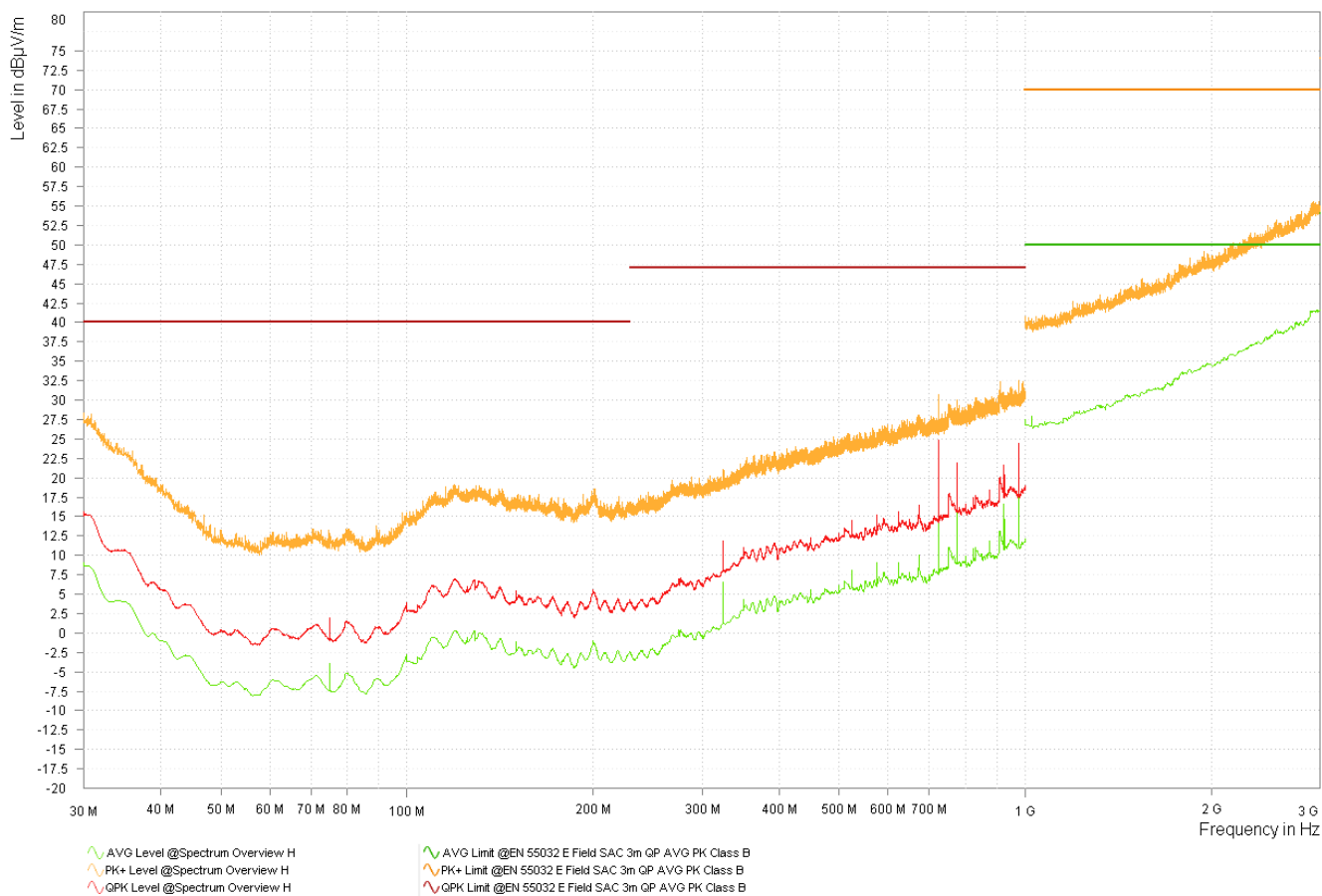
图 4-6. 型号 3 LMK3H0102-Q1 3.3V Y 轴频谱概述 - 水平
