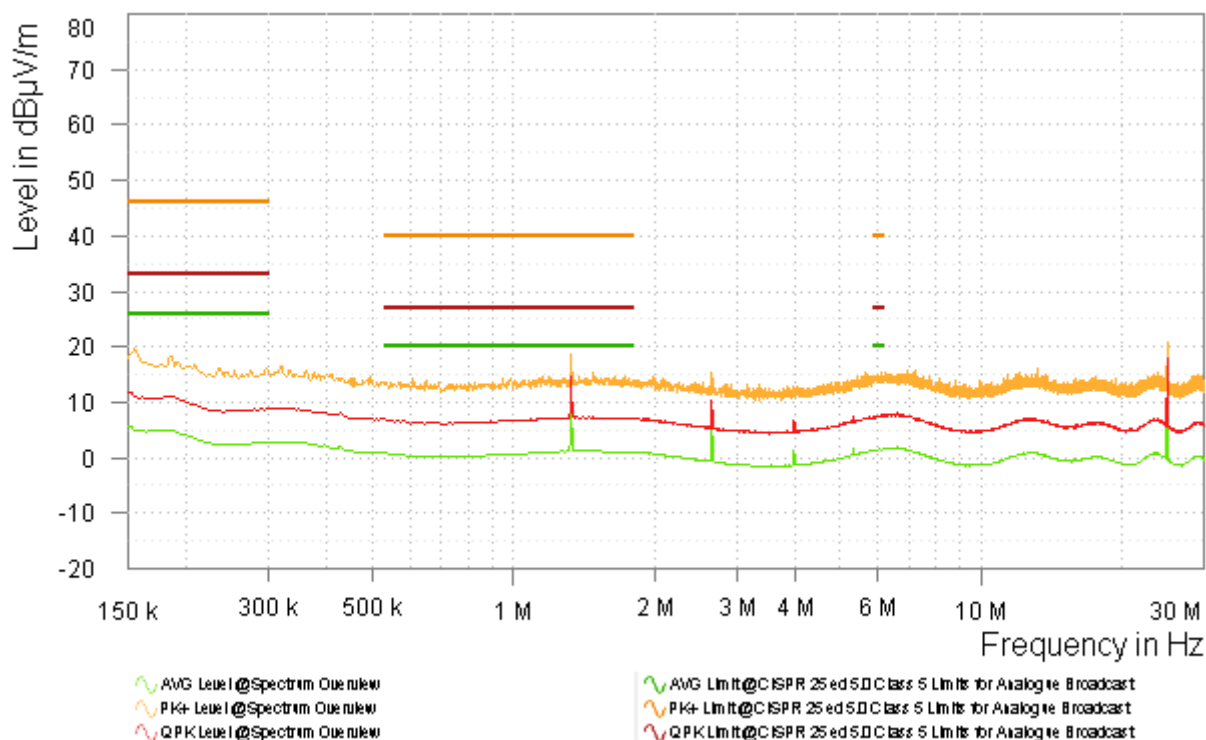
图 3-7. 型号 3 LMK3H0102-Q1 3.3V 频谱概述 - 单极
