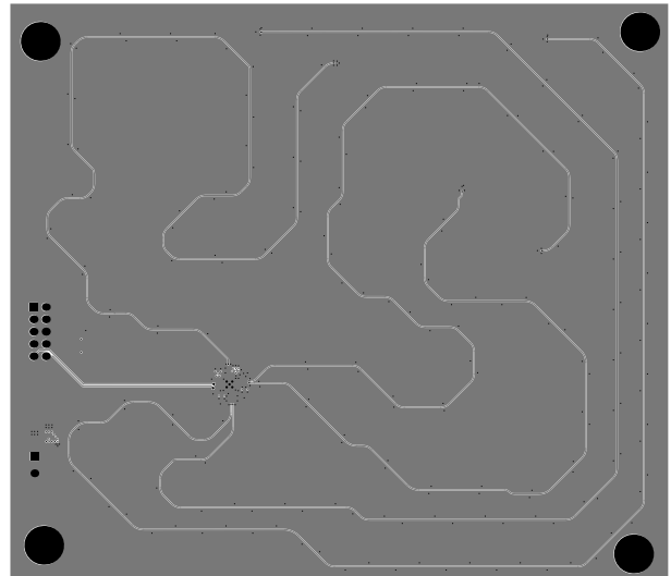
图 2-4. 型号 2 信号层布局
