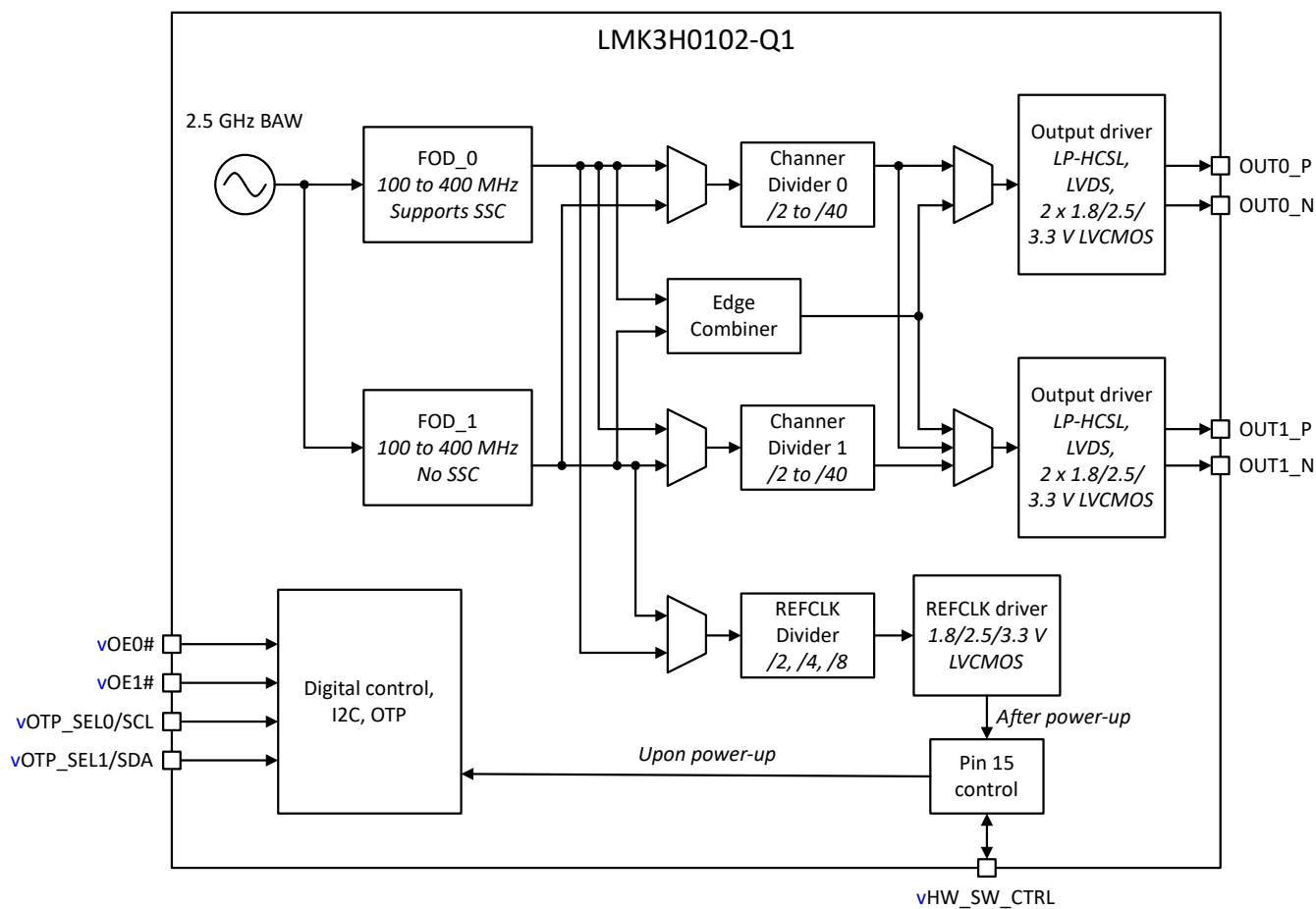
图 1-1. LMK3H0102-Q1 功能框图
