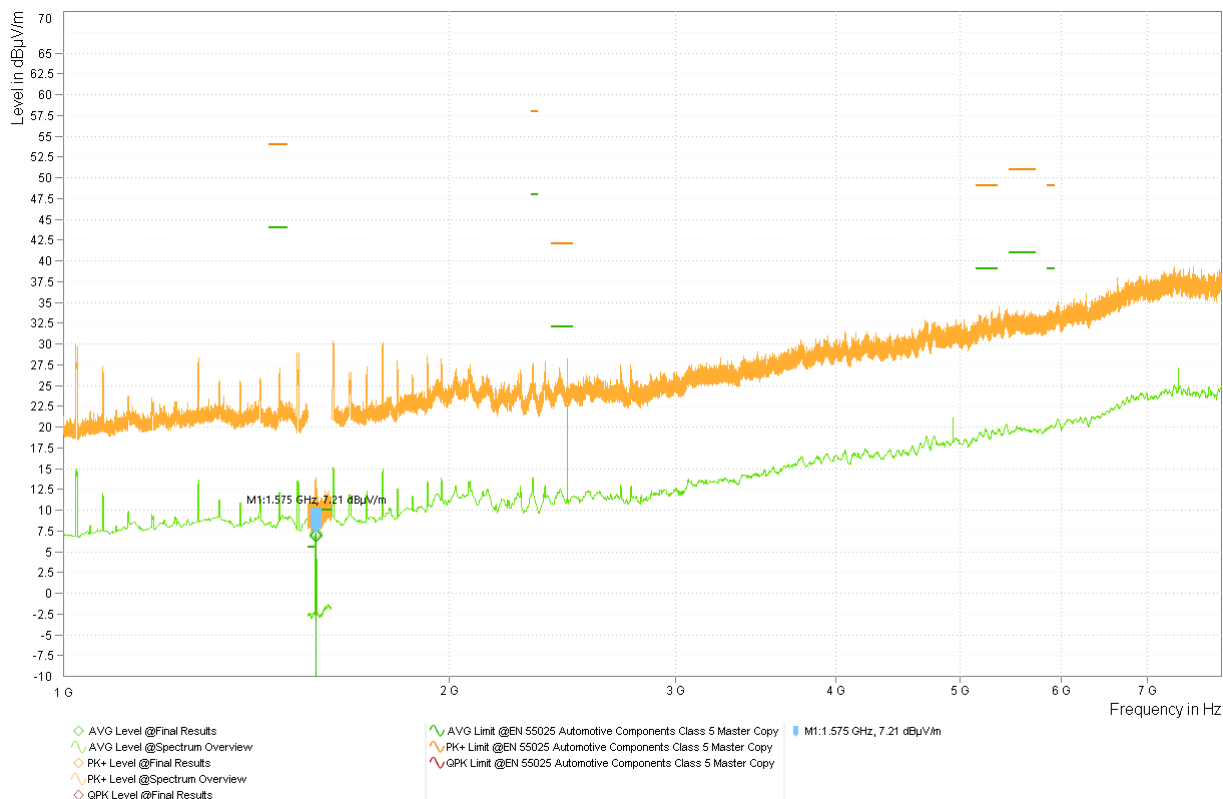
图 3-26. 型号 3 LMK3H0102-Q1 1.8V (带 -0.5% SSC) 频谱概述 - 喇叭
