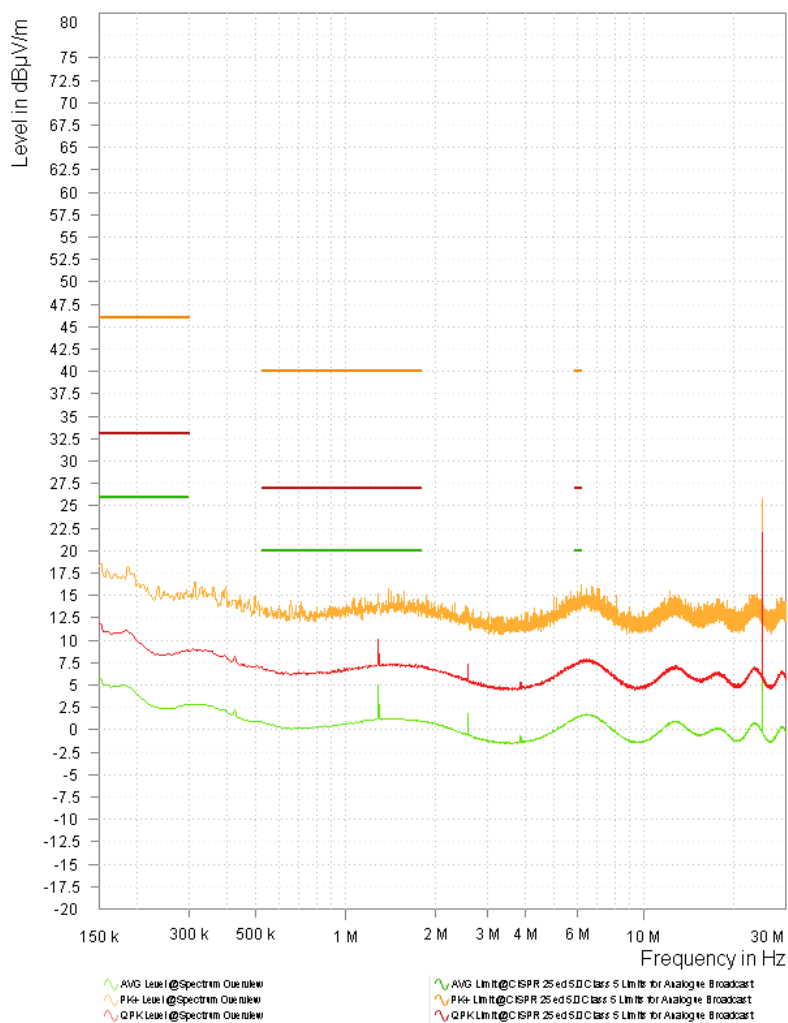
图 3-8. 型号 4 竞品振荡器 3.3V 频谱概述 - 单极
