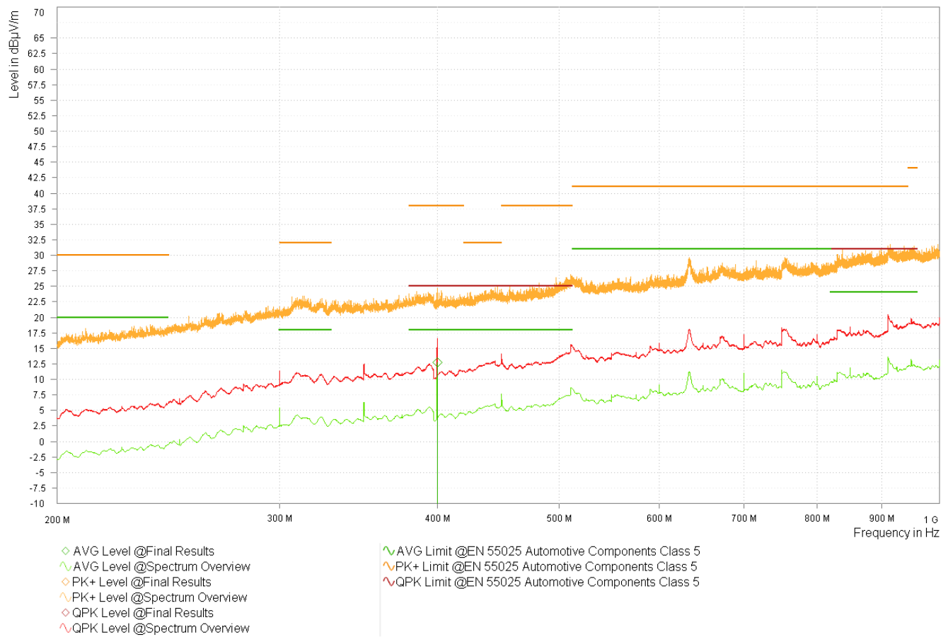
图 3-17. 型号 1 LMK3H0102-Q1 1.8V 频谱概述 - 对数周期
