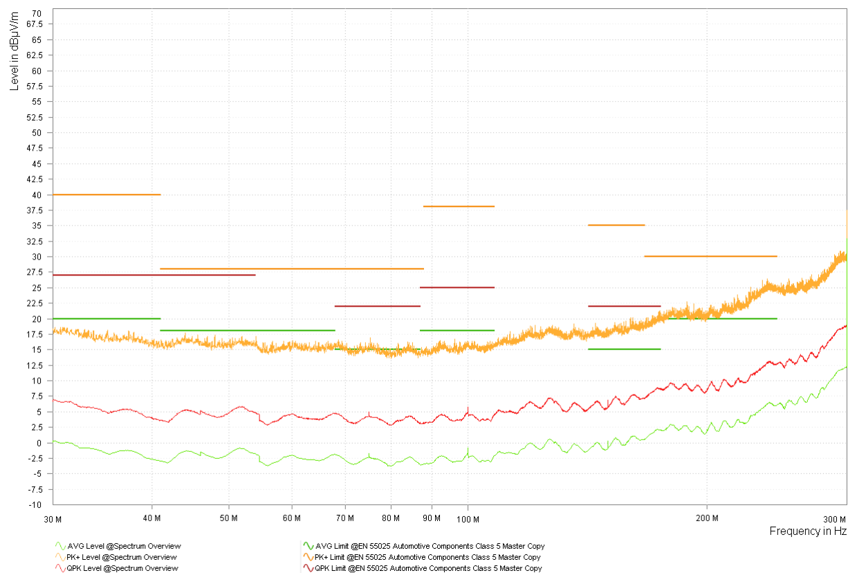
图 3-11. 型号 3 LMK3H0102-Q1 3.3V 频谱概述 - 双锥
