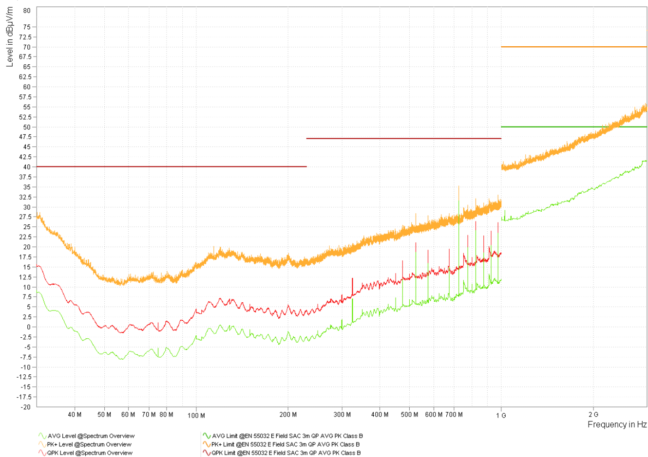
图 4-4. 型号 3 LMK3H0102-Q1 3.3V X 轴频谱概述
