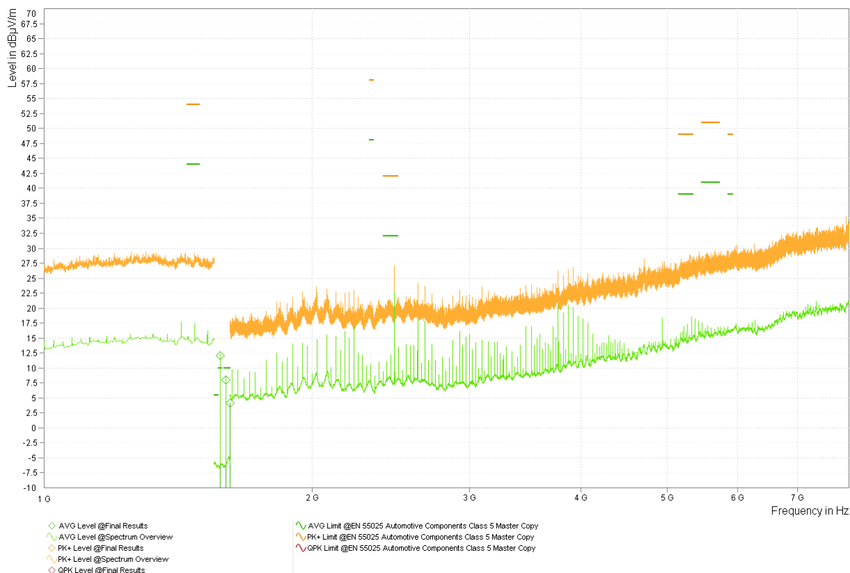
图 3-20. 型号 2 LMK3H0102-Q1 3.3V 频谱概述 - 喇叭
