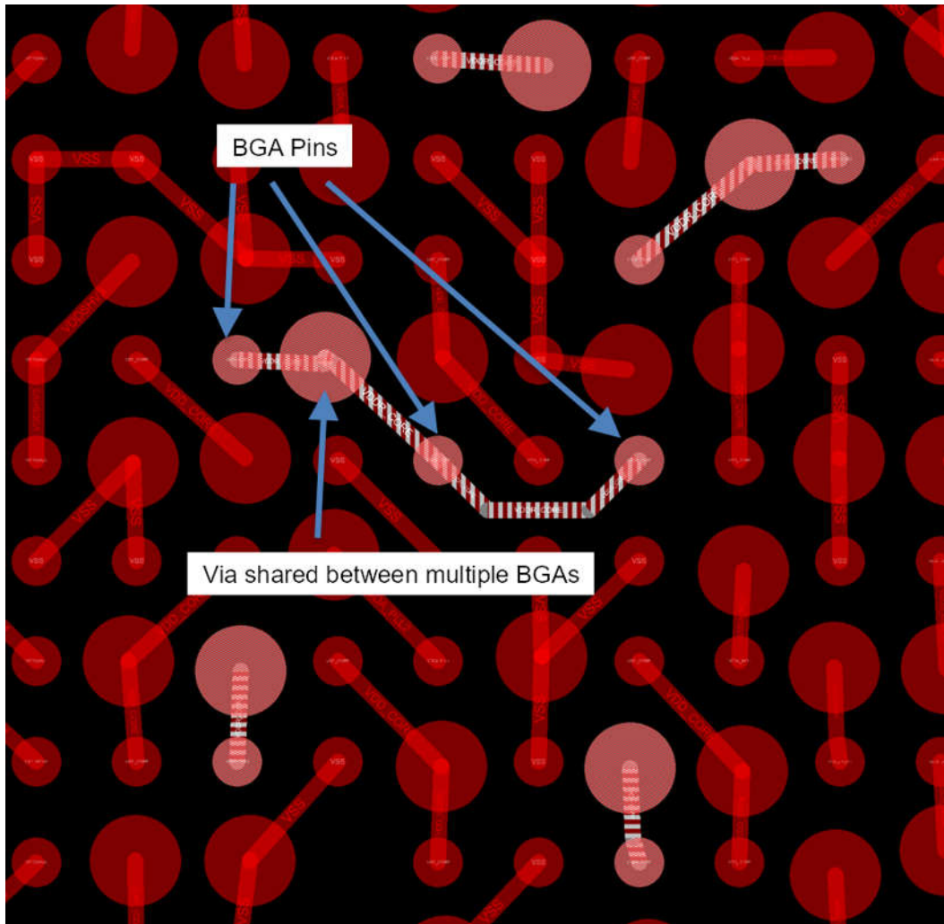
图 5-1. VDDR_CORE 域的过孔共享
