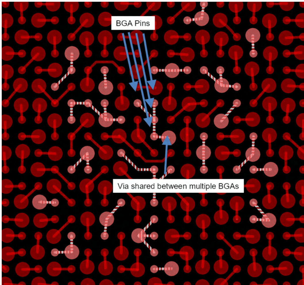
图 5-2. VSS 的过孔共享
