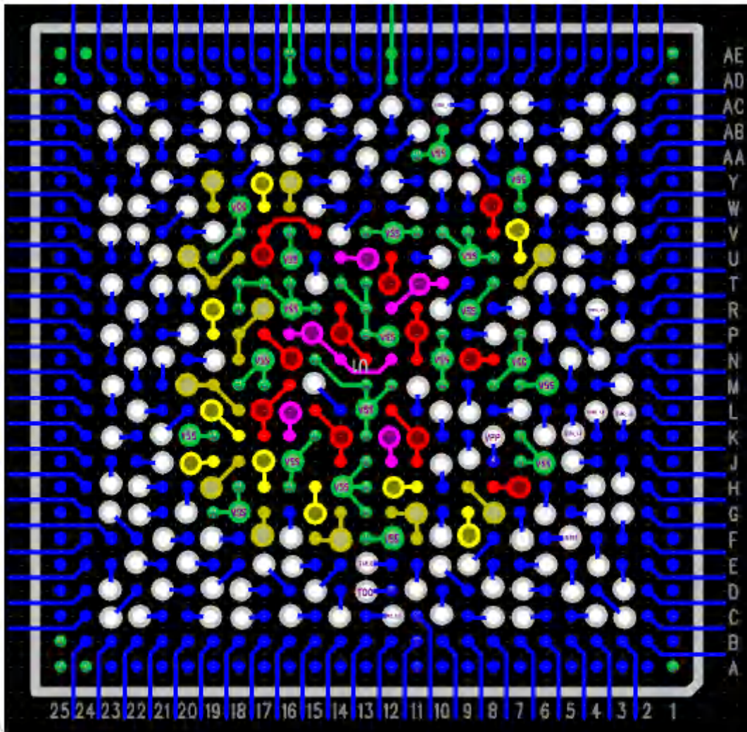
图 13-1. 具有完整信号和电源迂回布线的 AM62x
