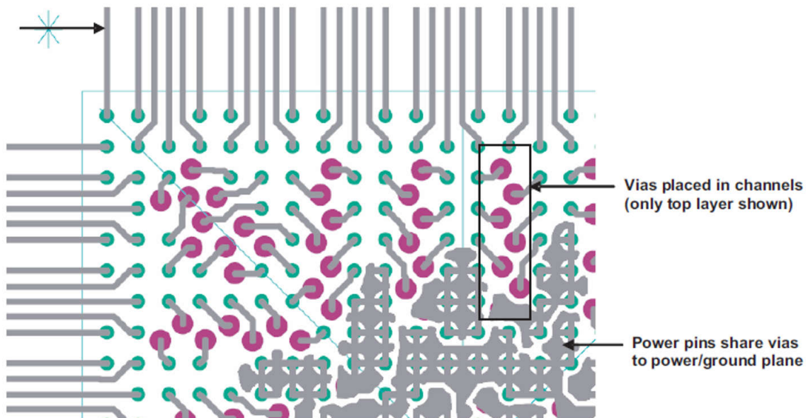
图 2-3. 过孔通道中的过孔
