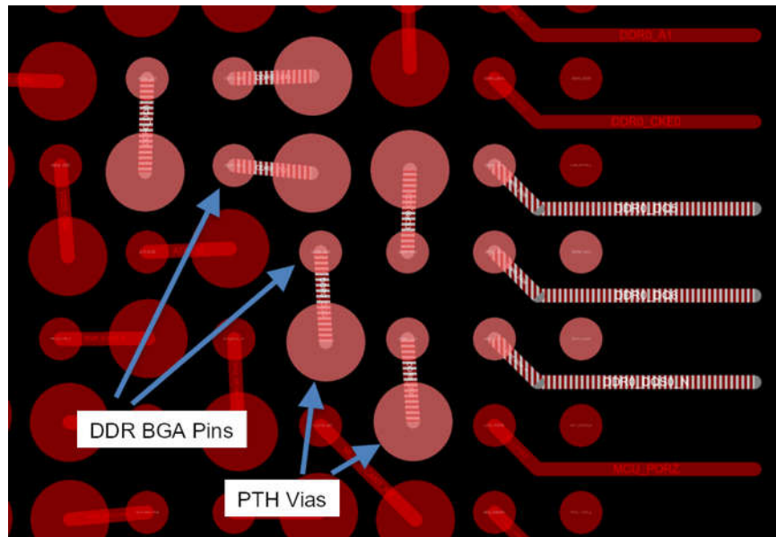
图 10-1. DDR 字节通道 0 迂回
