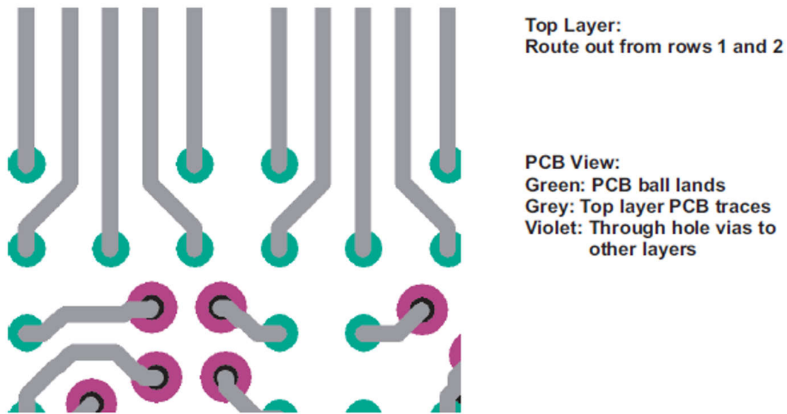
图 2-2. 布线外排
