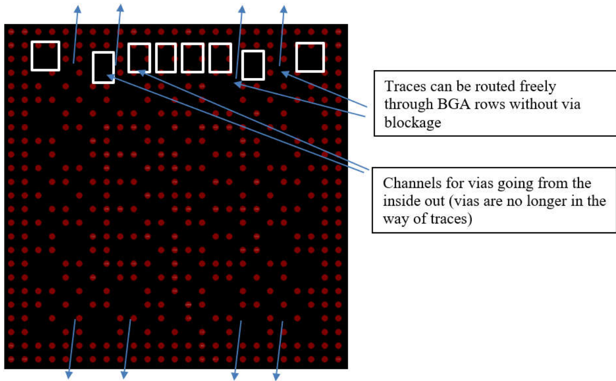
图 2-1. AM62x BGA 过孔通道阵列
