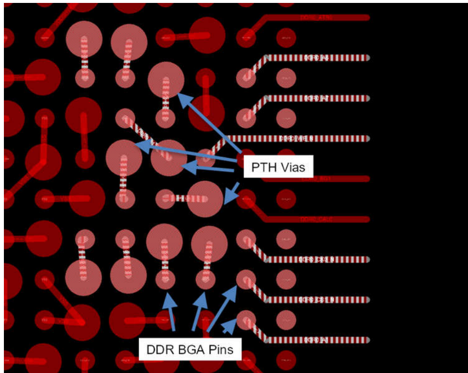
图 10-4. DDR 地址/命令迂回
