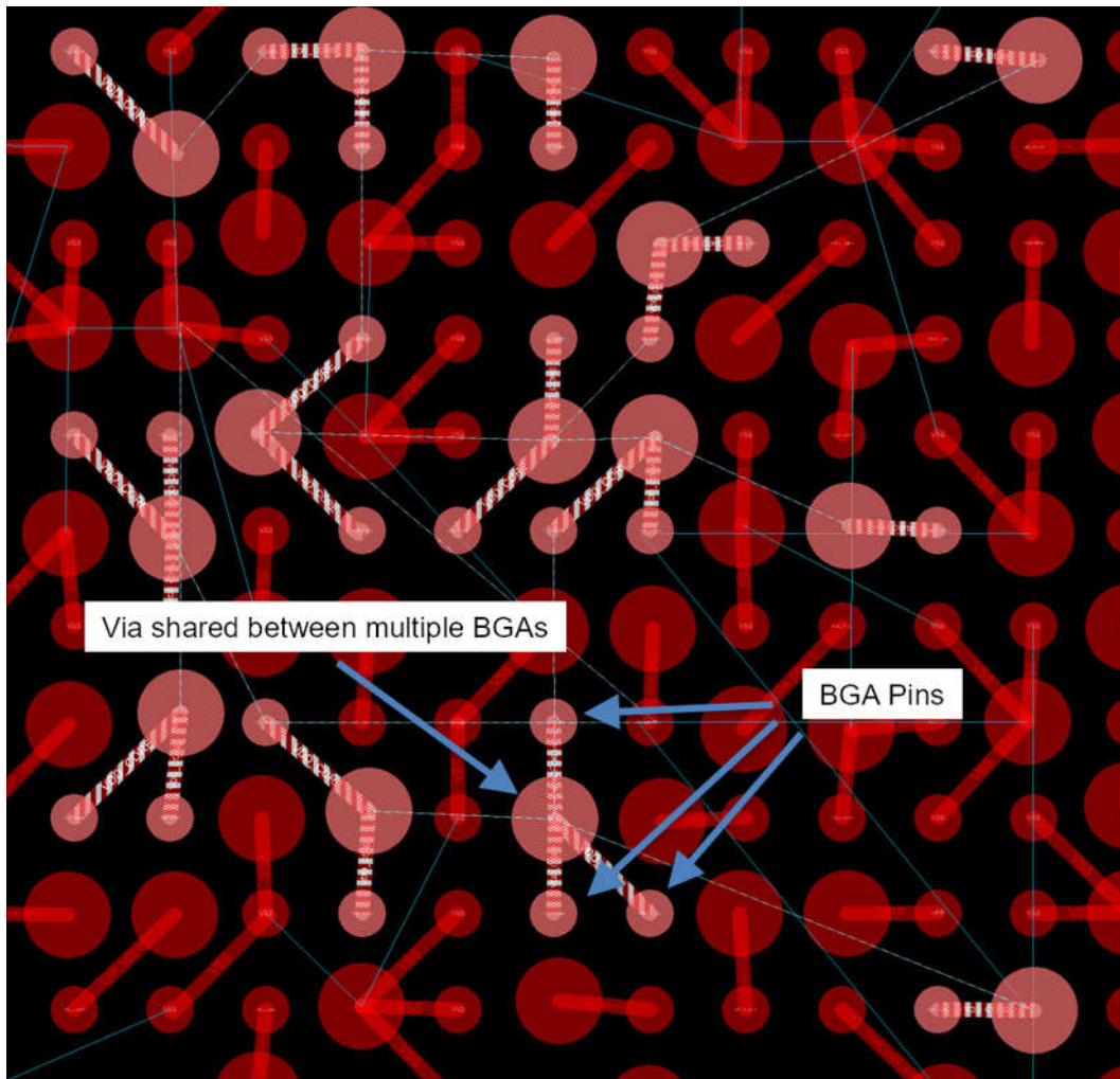
图 5-3. 合并的 VDD_CORE 和 VDDR_CORE 域的过孔共享
