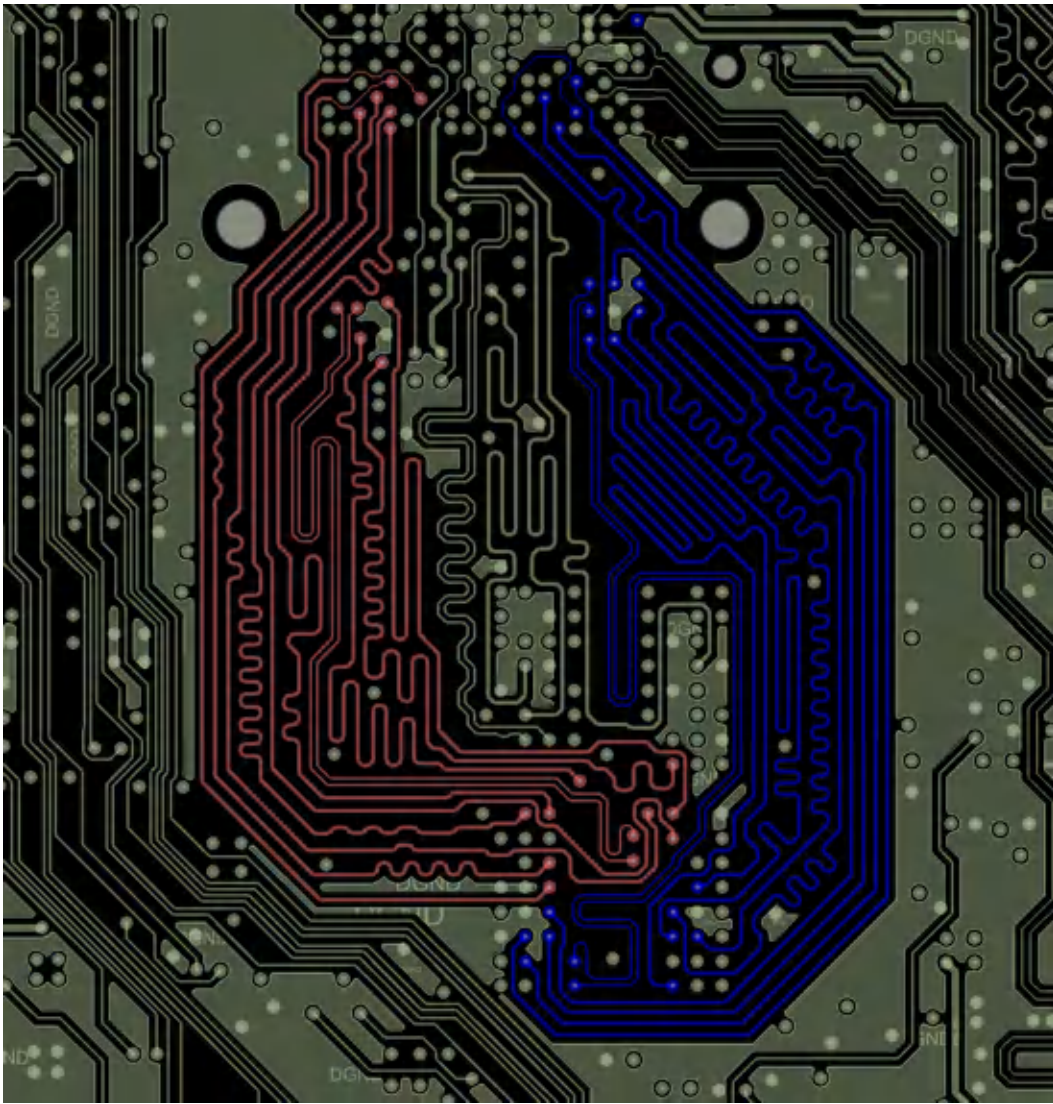
图 10-3. DDR 数据字节通道布线 ( 字节通道 0 - 左侧；字节通道 1 - 右侧 )
