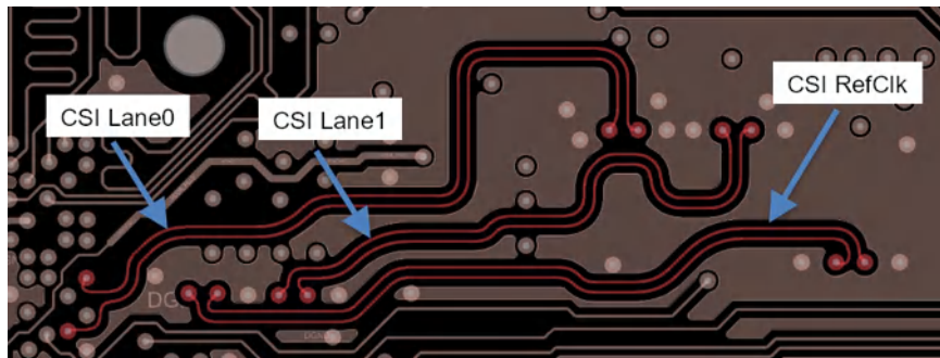
图 9-2. CSI 双路布线
