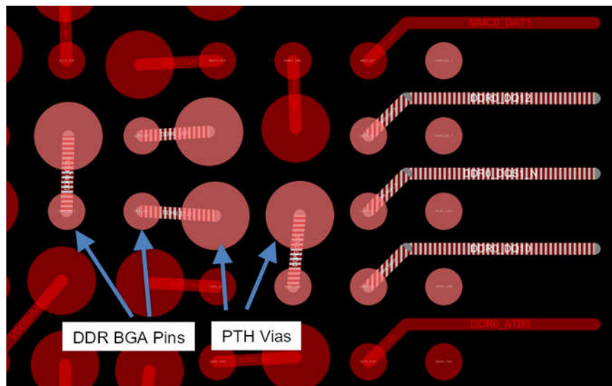
图 10-2. DDR 字节通道 1 迂回
