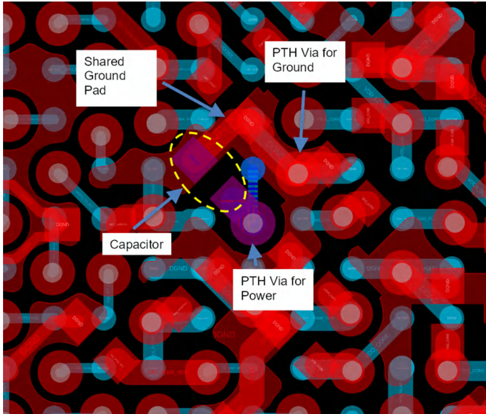
图 11-1. AM62 SK EVM CAP_VDDS0 输出电容器布局
