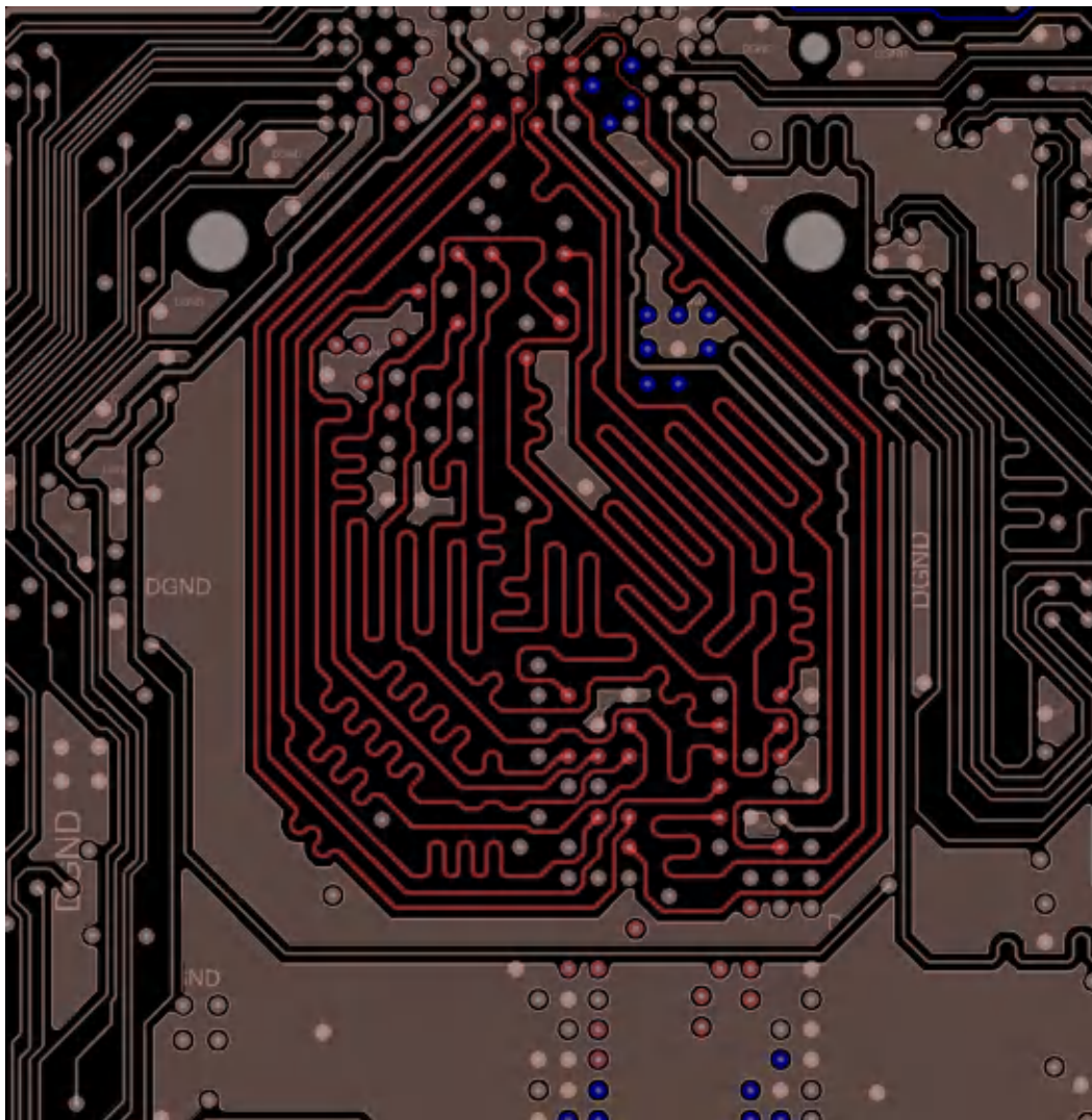
图 10-5. DDR4 地址、命令和时钟组布线
