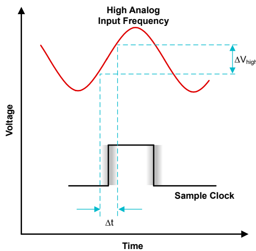
图 3-2. 低模拟输入频率与相同时间段内出现的相同采样时钟边沿 图 3-3. 高模拟输入频率与相同时间段内出现的相同采样时钟边沿
