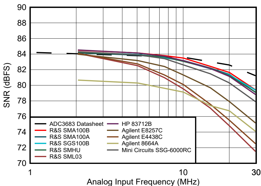
图 4-3. 在 25MSPS 和 +10dBm 条件下，以 -1dBFS 模拟输入信号运行 ADC 时，不同时钟信号源下 ADC3683 SNR 与 f_{in} 间的关系
