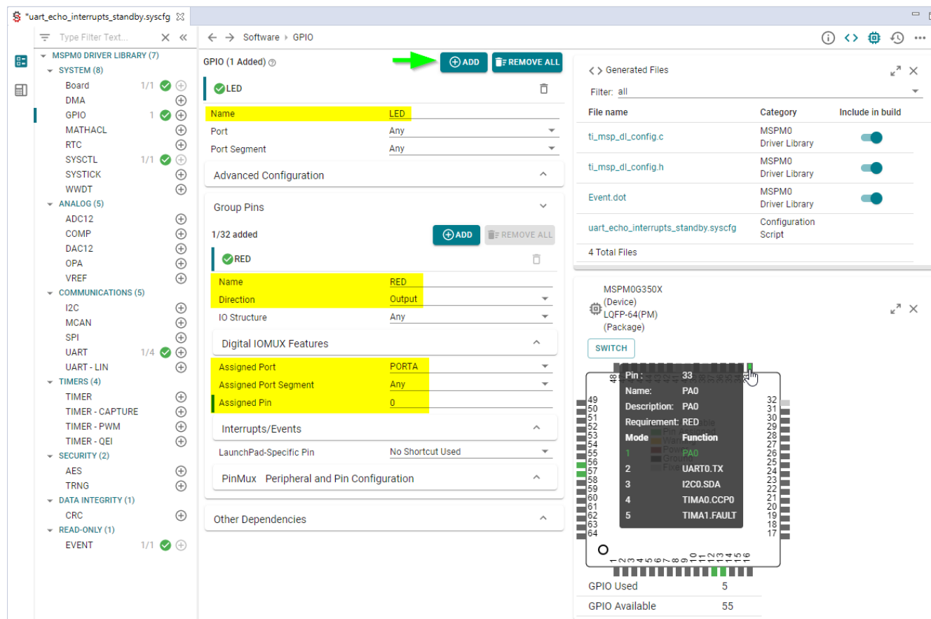
图 2-9. GPIO 配置
