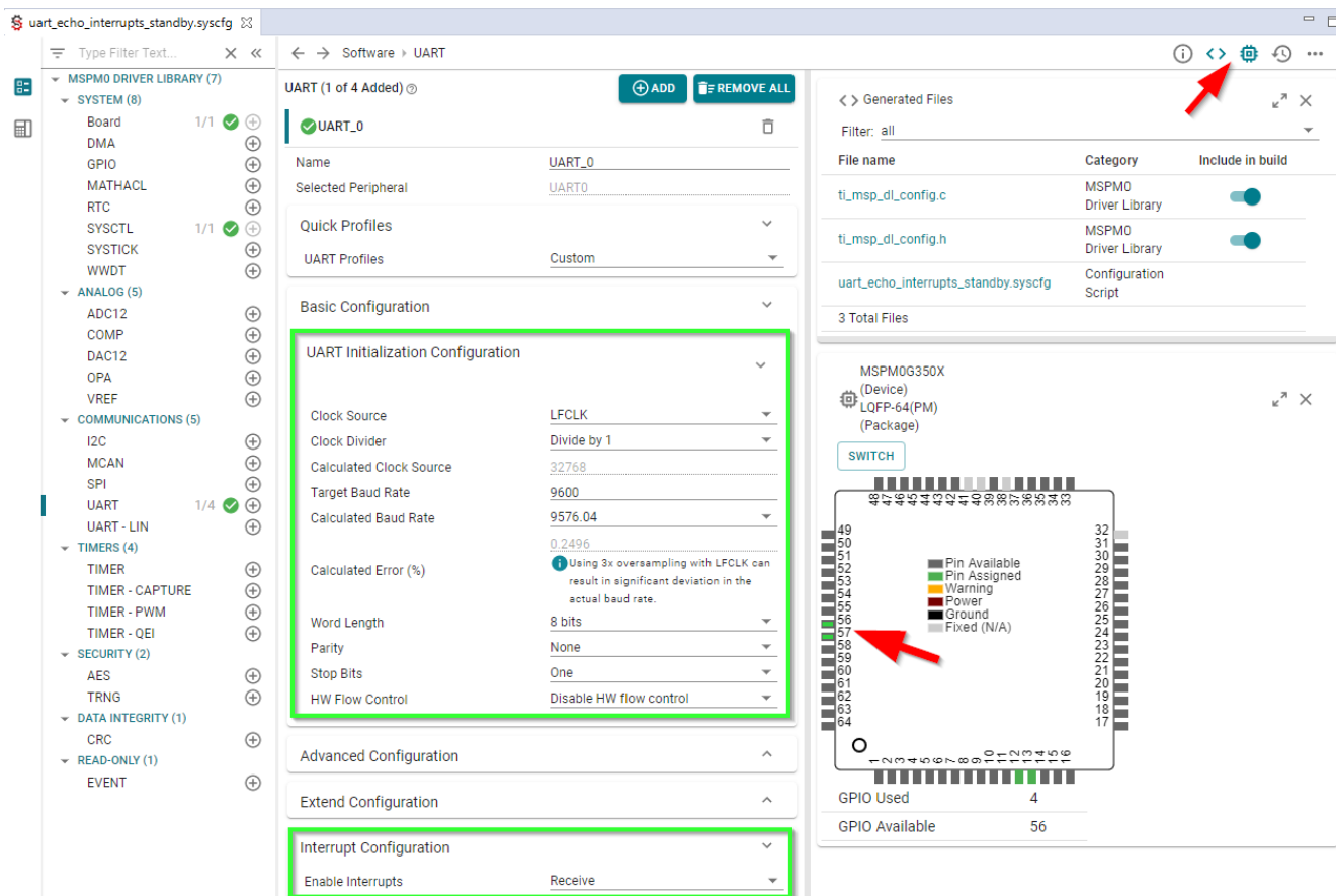
图 2-8. UART 配置
