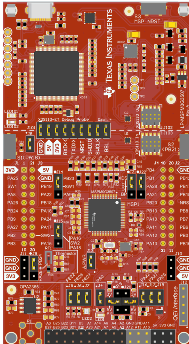
图 2-2. LP-MSPM0G3507 LaunchPad 开发套件
