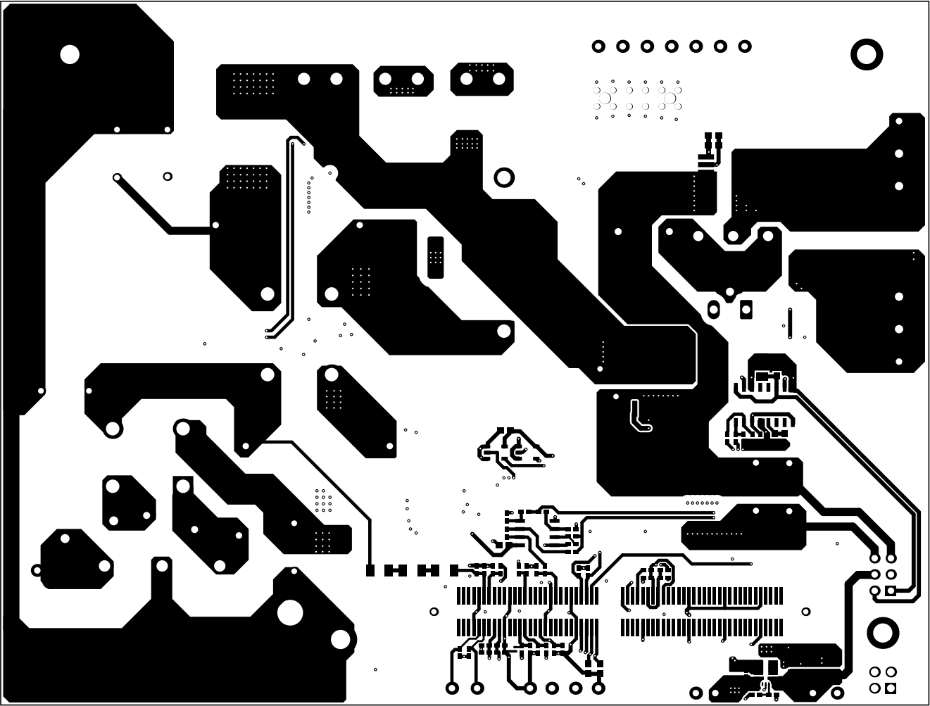
Top Layer
