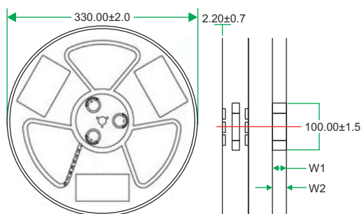
图 12-3. 卷盘规格
