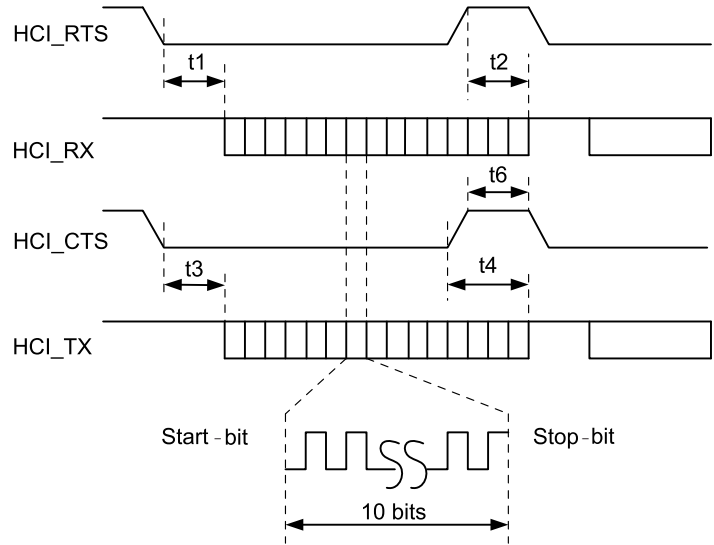
图 8-10. UART 时序图
