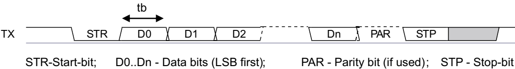
图 8-11. UART 数据帧
