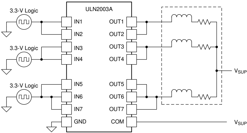
图 8-1. ULN2003A 器件用作感性负载驱动器
