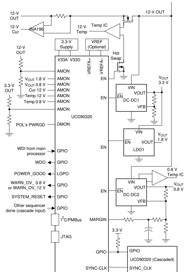
简化应用
