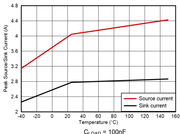
图 5-28. 峰值拉电流和灌电流
