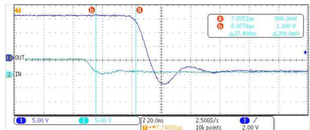
图 7-4. UCC57108 下降 (关断) 传播延迟
