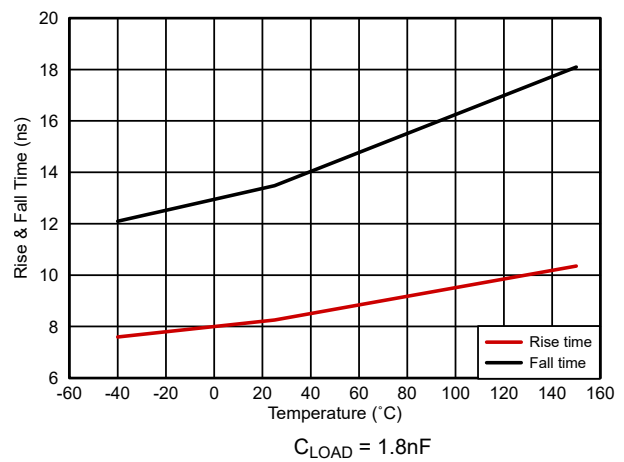
图 5-16. 输出上升和下降时间
