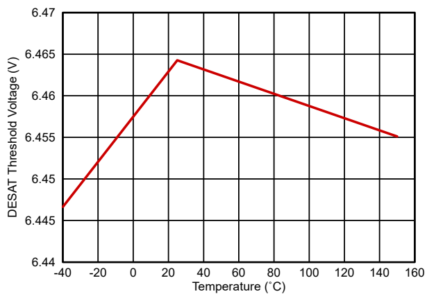
图 5-24. DESAT 阈值与温度间的关系
