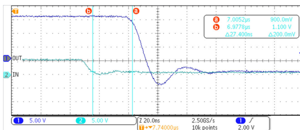
图 7-4. UCC57102Z-Q1 下降 ( 关断 ) 传播延迟
