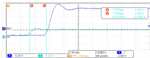
图 7-3. UCC57102Z-Q1 上升 ( 导通 ) 传播延迟
