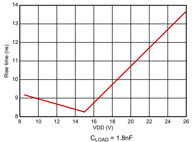
图 5-14. 输出上升时间
