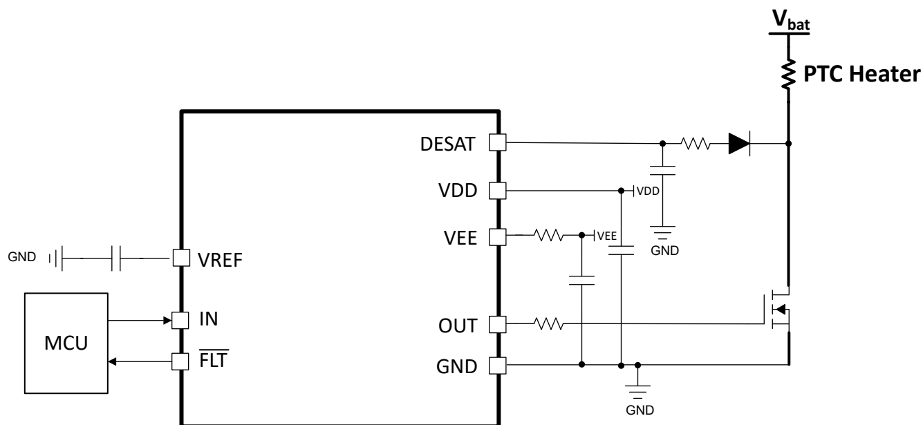
图 7-1. PTC 加热器应用中使用的 UCC57102Z
