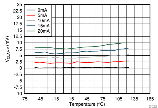
图 6-20. V_{CLAMP} vs Temperature
