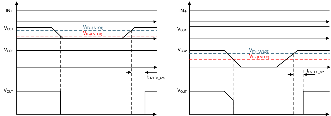
图 8-7. UVLO Functions
