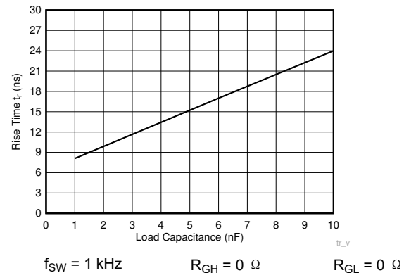
图 6-18. Rise Time vs Load Capacitance
