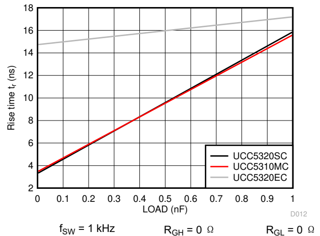
图 6-36. Rise Time vs Load Capacitance
