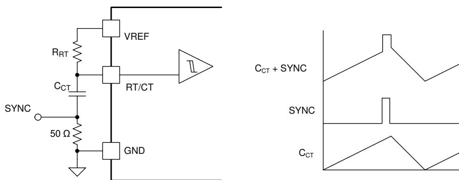
图 7-5. 振荡器同步电路
