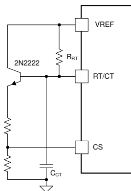
图 7-9. 电流模式 PWM 用作电压模式 PWM
