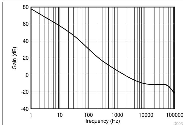
图 8-6. 转换器闭环波特图 - 增益
