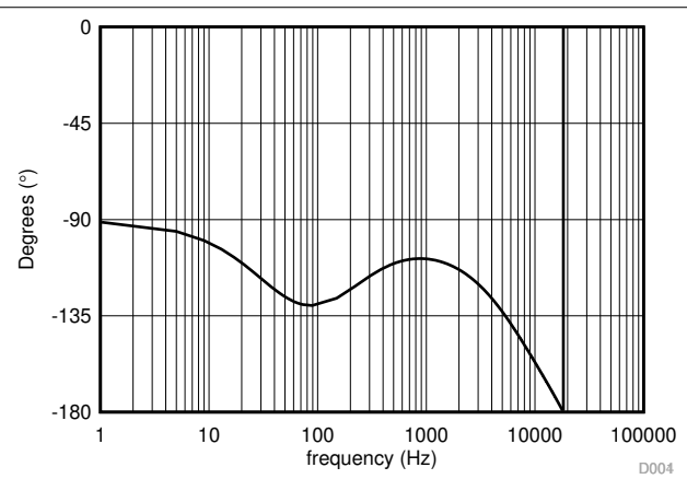
图 8-7. 转换器闭环波特图 - 相位
