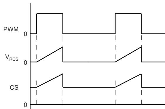
图 7-17. 带偏置的 CS 引脚电压
