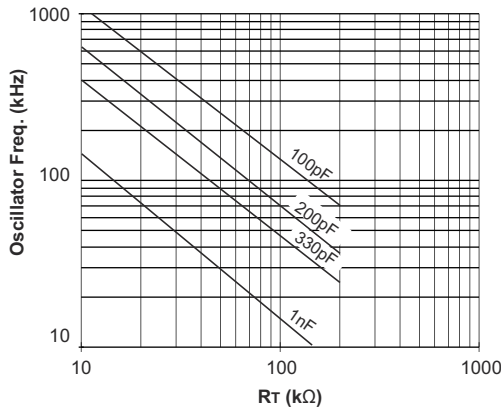
图 6-3. UCC3813-[0,1,2,4] : 振荡器频率与 R_{\text{T}} 和 C_{\text{T}} 间的关系
