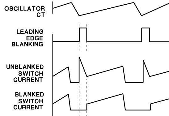
图 7-14. 具有前缘消隐的 UCCx813-x 电流检测波形
