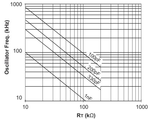
图 6-4. UCC3813-[3,5] : 振荡器频率与 R_{\text{T}} 和 C_{\text{T}} 间的关系
