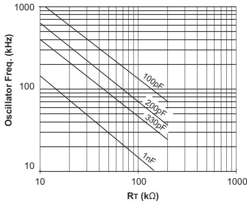
图 6-3. UCC3813-[0,1,2,4] : 振荡器频率与 R_T 和 C_T 间的关系
