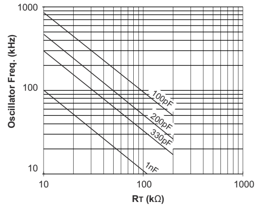
图 6-4. UCC3813-[3,5] : 振荡器频率与 R_T 和 C_T 间的关系
