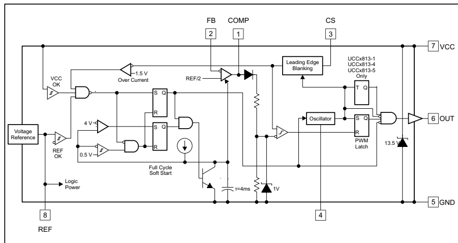
方框图
