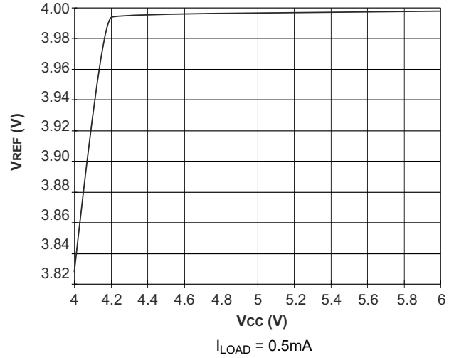
图 6-2. UCC3813-[3,5] : V_{\text{REF}} 与 V_{\text{CC}} 间的关系
