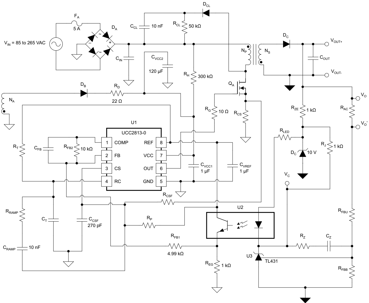
图 8-1. 典型应用电路图
