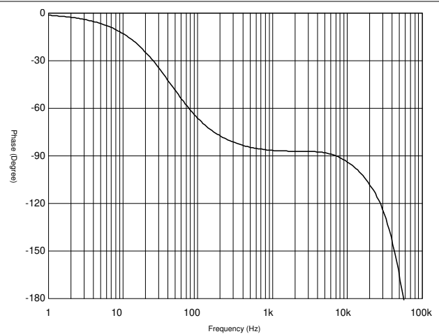
图 8-3. 转换器开环波德图：相位
