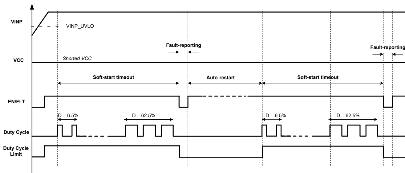
图 7-2. 短路输出下的软启动
