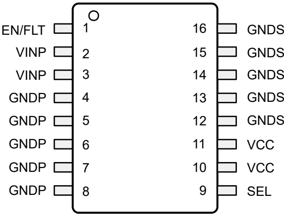
图 5-1. DHA SOIC 16 引脚封装，顶视图
