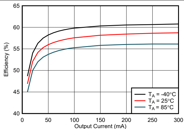
图 6-6. 效率与负载电流 ( I_{VCC} ) 间的关系 : V_{CC} = 5.0V , V_{INP} = 5.0V , C_{OUT2} = 22 \mu F
