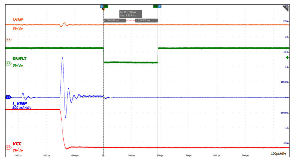
图 6-16. 输出短路运行: VINP = 5.0V
