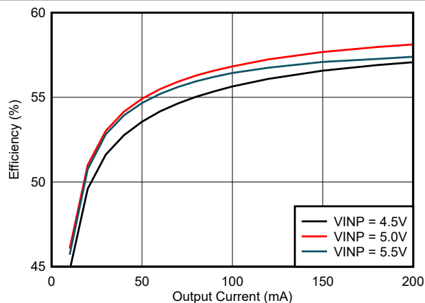
图 6-7. 效率与负载电流 ( I_{VCC} ) 间的关系: V_{CC} = 5.5V , T_A = 25^\circ C , C_{OUT2} = 22 \mu F
