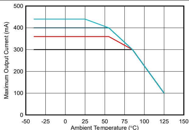
图 6-3. 最大输出电流与环境温度间的关系 : V_{CC} = 5.0V , C_{OUT2} = 22 \mu F
