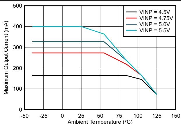
图 6-4. 最大输出电流与环境温度间的关系 : V_{CC} = 5.5V , C_{OUT2} = 22 \mu F
