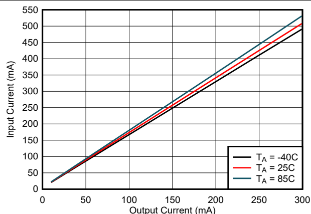
图 6-9. 输入电流 ( I_{VINP} ) 与负载电流 ( I_{VCC} ) 间的关系: V_{CC} = 5.0V , V_{INP} = 5.0V , C_{OUT2} = 22 \mu F
