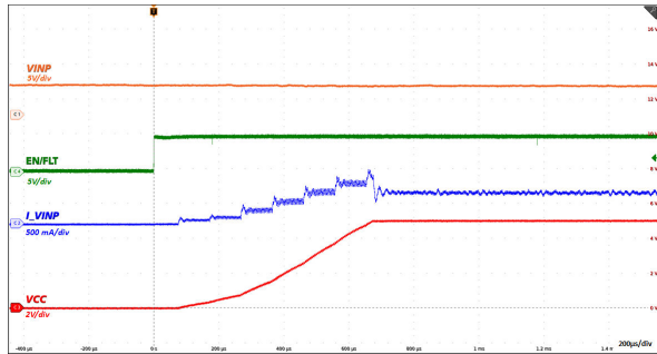
图 6-13. 通过 EN/FLT 从低电平到高电平启动: VINP = 5.0V, VCC = 5.0V, 18Ω 负载
