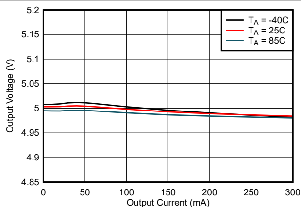
图 6-11. 输出电压调节 ( V_{VCC} ) 与负载电流 ( I_{VCC} ) 间的关系: V_{CC} = 5.0V , V_{INP} = 5.0V , C_{OUT2} = 22 \mu F
