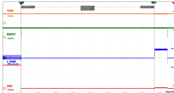
图 6-17. 短路输出下的自动重启操作: VINP = 5.0V
