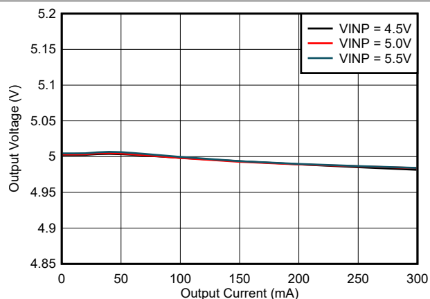
图 6-10. 输出电压调节 ( V_{VCC} ) 与负载电流 ( I_{VCC} ) 间的关系: V_{CC} = 5.0V , T_A = 25^\circ C , C_{OUT2} = 22 \mu F
