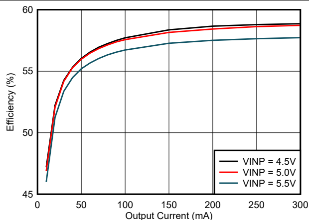
图 6-5. 效率与负载电流 ( I_{VCC} ) 间的关系 : V_{CC} = 5.0V , T_A = 25^\circ C , C_{OUT2} = 22 \mu F
