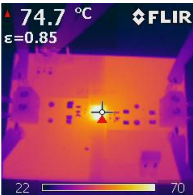
图 8-3. UCC33420-Q1 热像图 : V_{INP} = 5.0V , V_{CC} = 5.0V , P_{Out} = 1.5W
