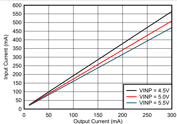
图 6-8. 输入电流 ( I_{VINP} ) 与负载电流 ( I_{VCC} ) 间的关系: V_{CC} = 5.0V , T_A = 25^\circ C , C_{OUT2} = 22 \mu F
