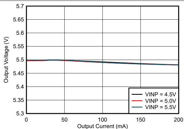
图 6-12. 输出电压调节 ( V_{VCC} ) 与负载电流 ( I_{VCC} ) 间的关系: V_{CC} = 5.5V , T_A = 25^\circ C , C_{OUT2} = 22 \mu F
