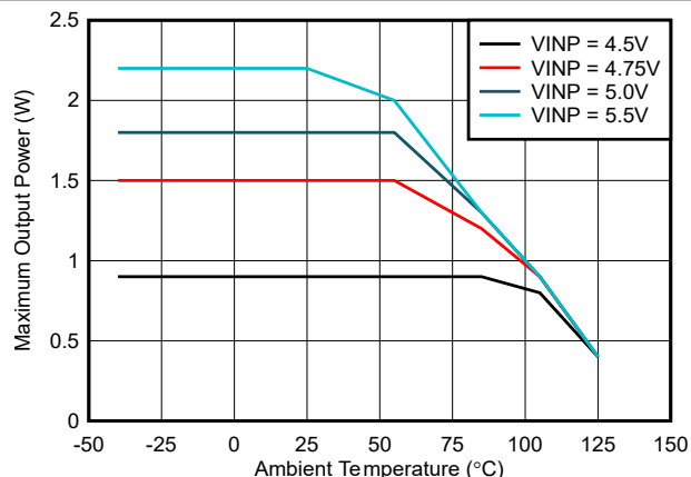
图 6-2. 最大输出功率与环境温度间的关系 : V_{CC} = 5.5V , C_{OUT2} = 22 \mu F
