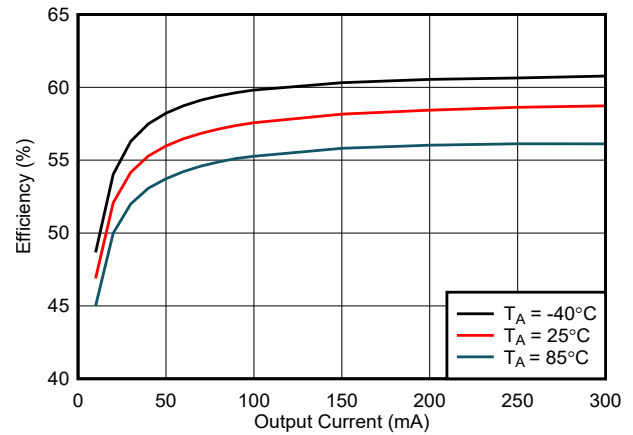
图 6-6. 效率与负载电流 ( I_{VCC} ) 间的关系 : V_{CC} = 5.0V , V_{INP} = 5.0V , C_{OUT2} = 22 \mu F
