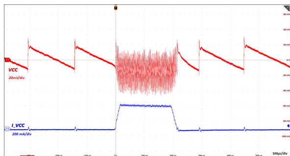
图 6-15. 负载瞬态 : VINP = 5.0V , VCC = 5.0V , C OUT2 = 22 µF , I VCC = 0mA - 300mA - 0mA
