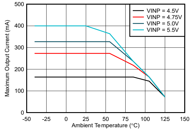
图 6-4. 最大输出电流与环境温度间的关系 : V_{CC} = 5.5V , C_{OUT2} = 22 \mu F
