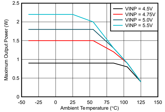
图 6-2. 最大输出功率与环境温度间的关系 : V_{CC} = 5.5V , C_{OUT2} = 22 \mu F
