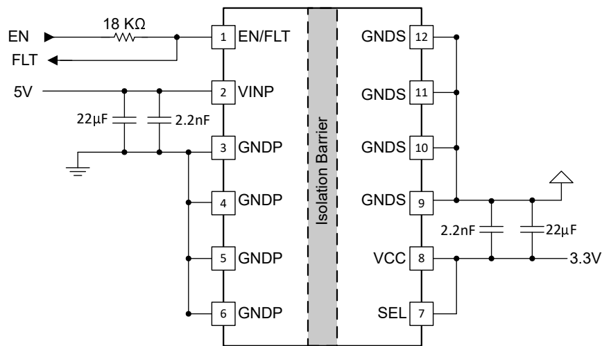
图 7-1. 典型应用
