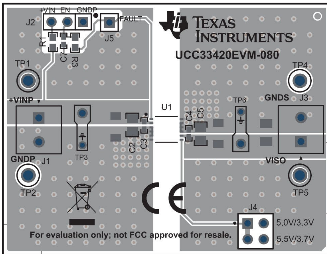
图 7-2. 布局示例
