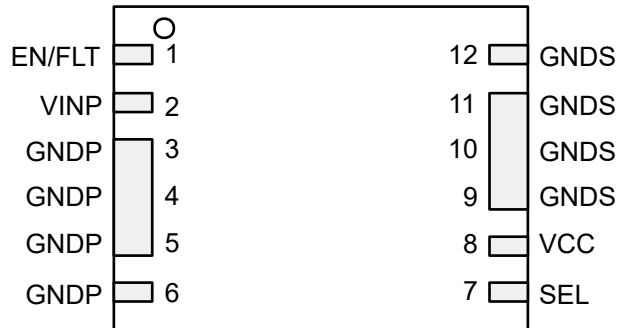
图 4-1. VSON-FCRL12 引脚封装，顶视图
