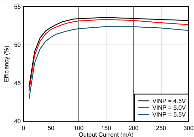
图 6-9. 效率与负载电流 ( I_{VCC} ) 间的关系: V_{CC} = 5.0V , T_A = 25^\circ C , C_{OUT2} = 22\mu F
