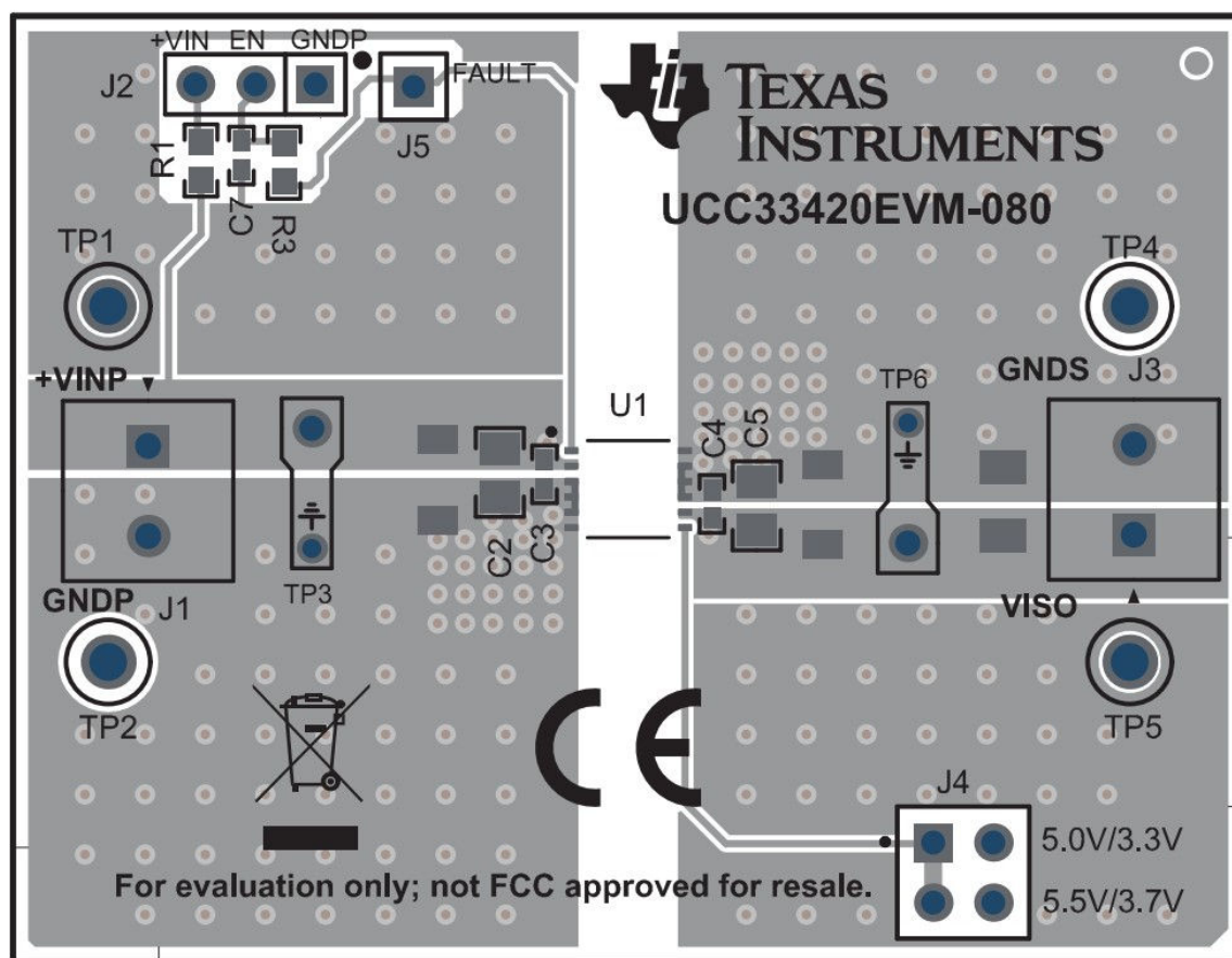
图 8-2. 布局示例
