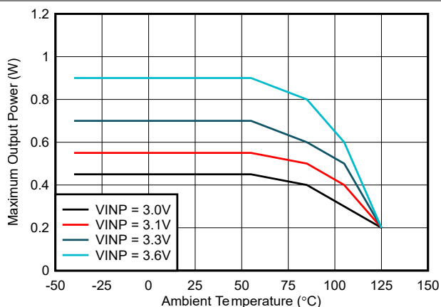
图 6-4. 最大输出功率与环境温度间的关系 : V_{CC} = 5.5V , C_{OUT2} = 22\mu F
