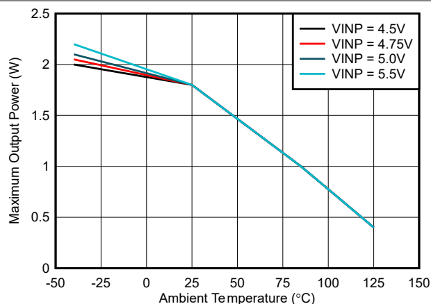
图 6-3. 最大输出功率与环境温度间的关系 : V_{CC} = 5.5V , C_{OUT2} = 22\mu F
