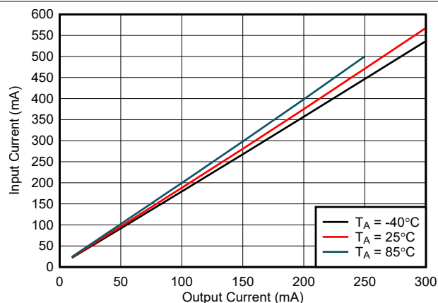
图 6-16. 输入电流 ( I_{VINP} ) 与负载电流 ( I_{VCC} ) 间的关系: V_{CC} = 5.0V , V_{INP} = 5.0V , C_{OUT2} = 22 \mu F
