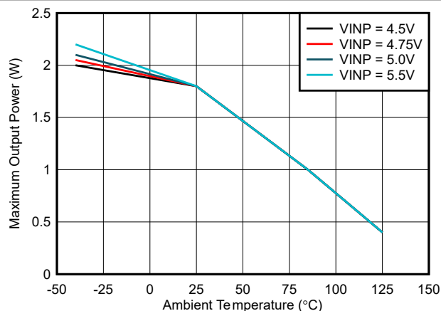
图 6-1. 最大输出功率与环境温度间的关系 : V_{CC} = 5.0V , C_{OUT2} = 22\mu F
