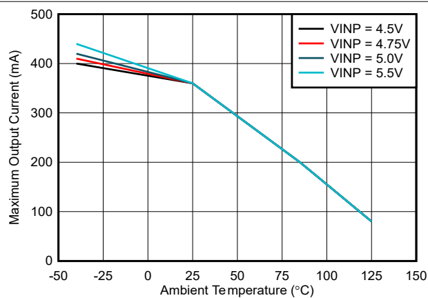
图 6-5. 最大输出电流与环境温度间的关系 : V_{CC} = 5.0V , C_{OUT2} = 22\mu F
