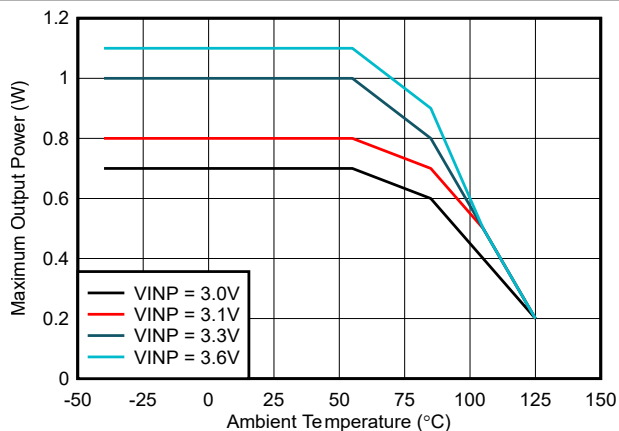
图 6-2. 最大输出功率与环境温度间的关系 : V_{CC} = 5.0V , C_{OUT2} = 22\mu F
