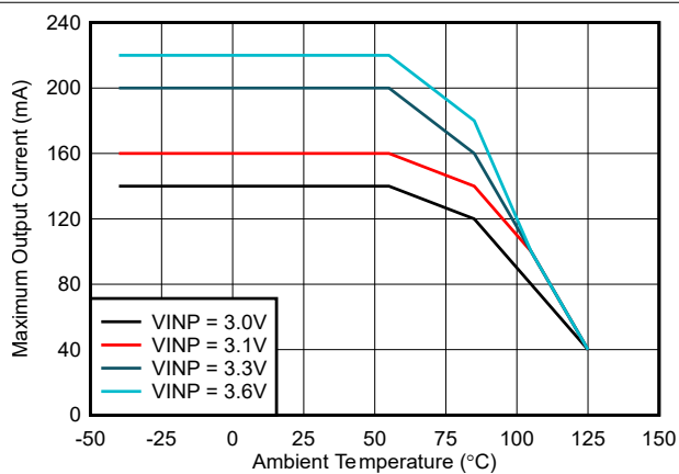
图 6-6. 最大输出电流与环境温度间的关系 : V_{CC} = 5.0V , C_{OUT2} = 22\mu F
