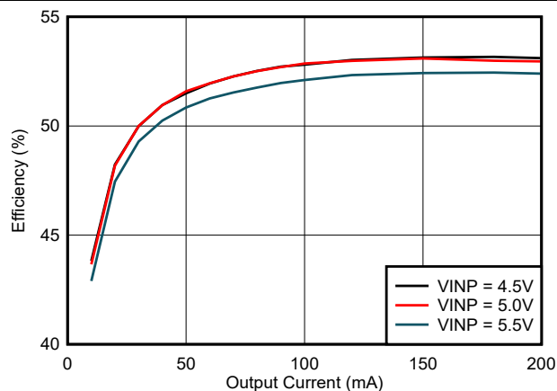
图 6-11. 效率与负载电流 ( I_{VCC} ) 间的关系: V_{CC} = 5.5V , T_A = 25^\circ C , C_{OUT2} = 22\mu F
