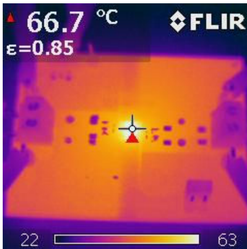
图 10-2. UCC33020 热像图 : V_{INP} = 5.0V , V_{CC} = 5.0V , P_{Out} = 1.0W
