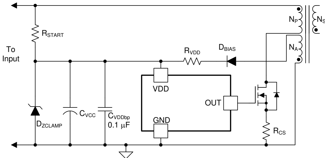
图 8-1. VDD Protection
