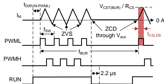
图 25. PWM Pattern in ABM
