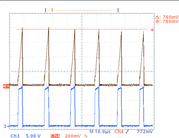
图 8-5. EMI Dithering
