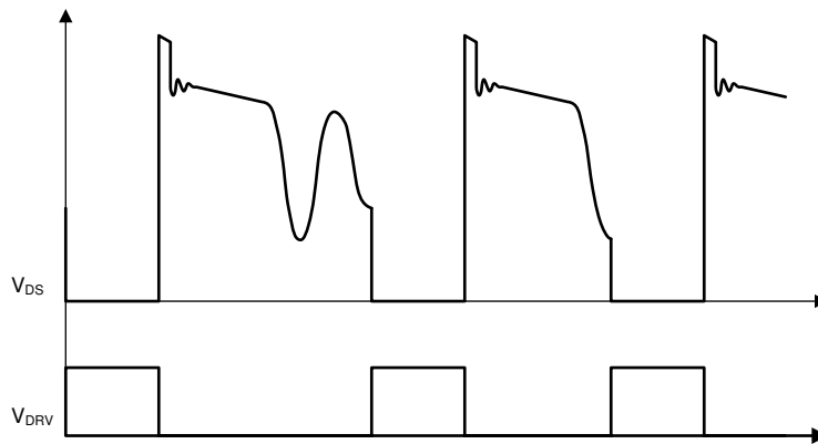
图 7-1. Valley-Skipping Mode
