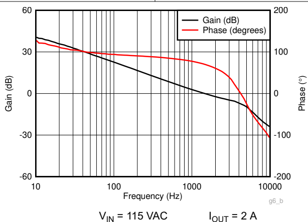
图 8-11. Bode Plot
