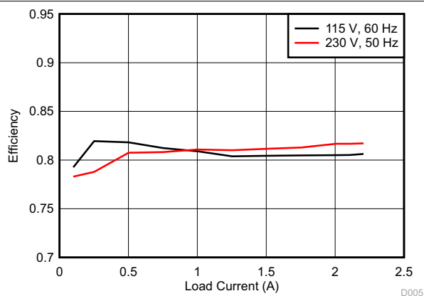
图 8-6. Efficiency
