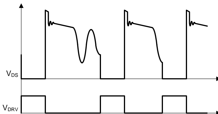
图 22. Valley-Skipping Mode
