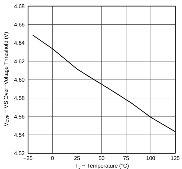
Figure 11. 过压 阈值与 温度间的关系
