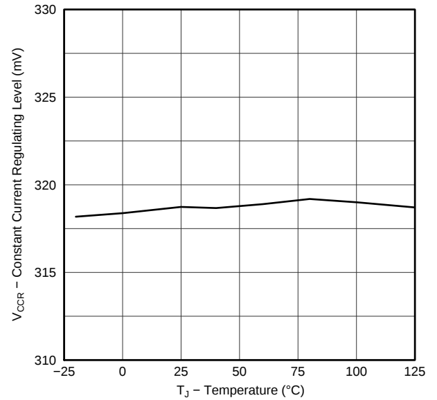
Figure 6. 恒定电流调节电平与 温度间的关系
