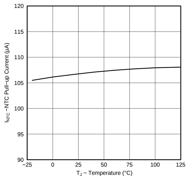
Figure 10. NTC 上拉 电流与 温度间的关系
