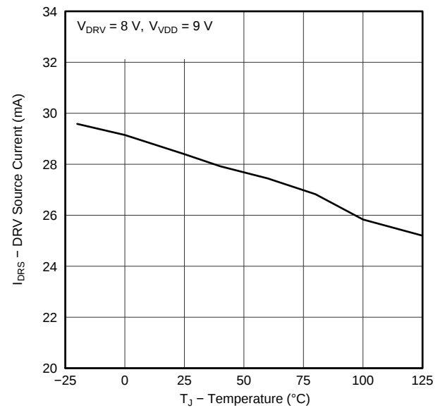
Figure 8. DRV 源 电流与 温度间的关系
