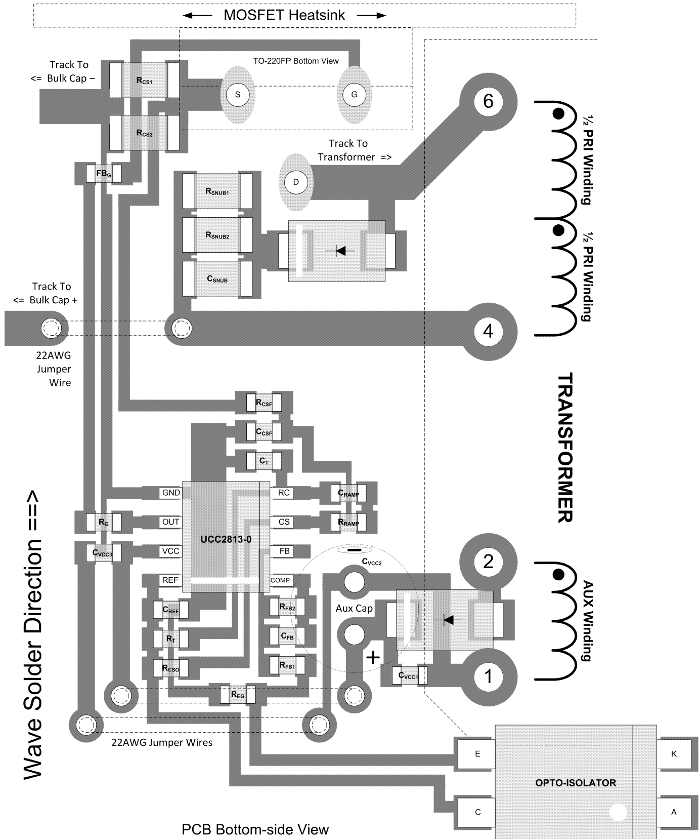
图 8-12 单层 PCB 的 UCC2813-0 布局示例
