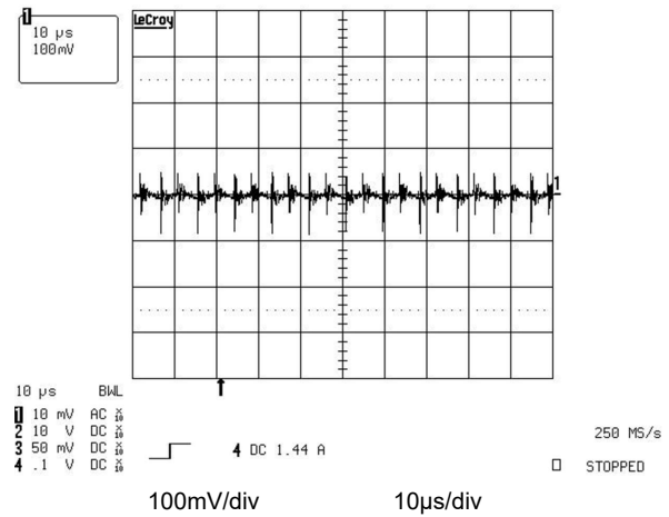
图 8-9. 满载条件下的输出电压纹波
