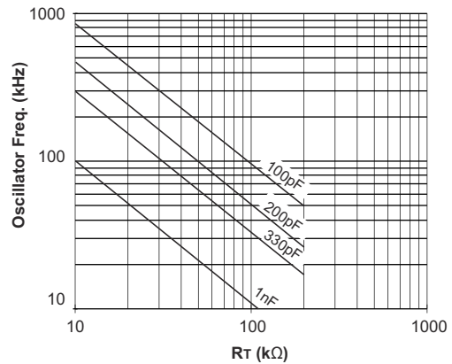
图 6-4. UCC2813-[3,5]-Q1 : 振荡器频率与 R_T 和 C_T 间的关系
