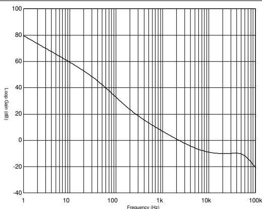
图 8-4. 转换器闭环波特图：增益
