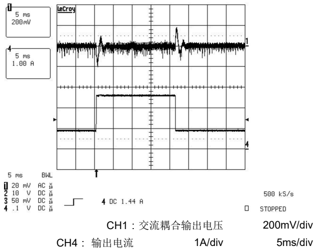
图 8-8. 0.9A 至 2.7A 负载瞬态期间的输出电压
