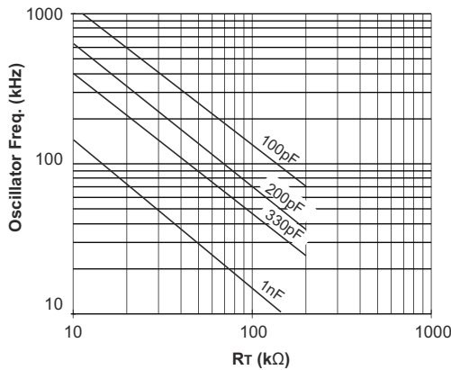
图 6-3. UCC2813-[0,1,2,4]-Q1 : 振荡器频率与 R_T 和 C_T 间的关系
