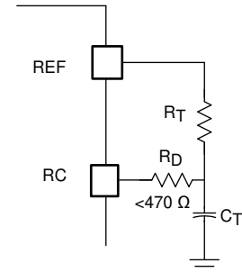
Copyright © 2016, Texas Instruments Incorporated 图 7-11. 电路产生受控的最大占空比
