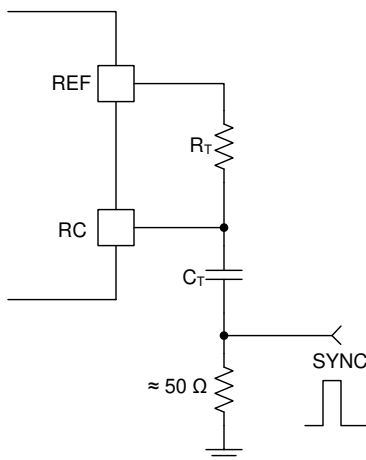
图 7-9. 同步振荡器
