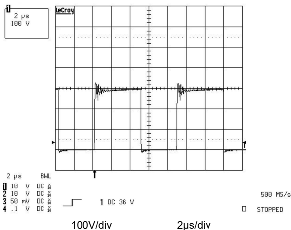
图 8-7. 120V 交流输入下的初级侧 MOSFET 漏源电压
