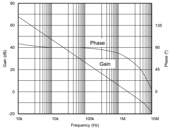
图 6-1. 误差放大器增益与相位响应
