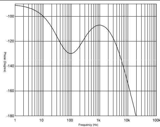
图 8-5. 转换器闭环波特图：相位
