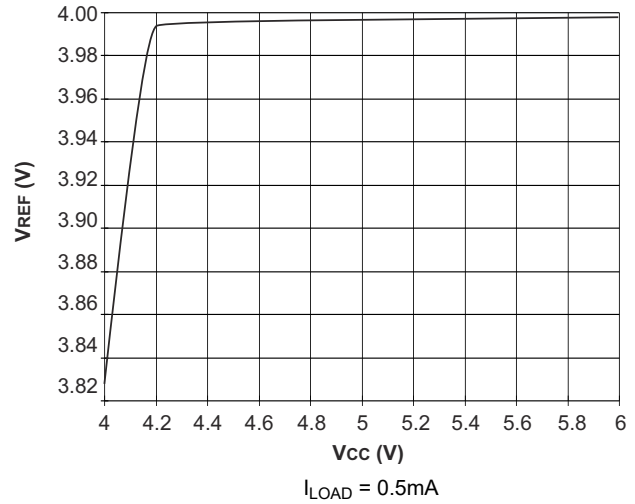
图 6-2. UCC2813-[3,5]-Q1 : V_{REF} 与 V_{CC} 间的关系
