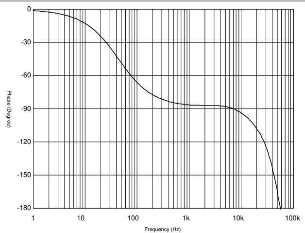
图 8-3. 转换器开环波特图：相位
