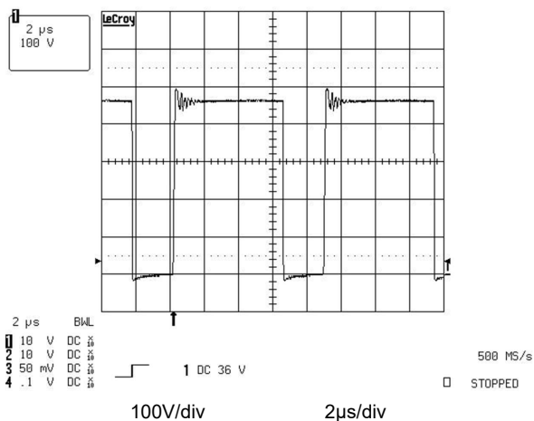
图 8-6. 240V 交流输入下的初级侧 MOSFET 漏源电压
