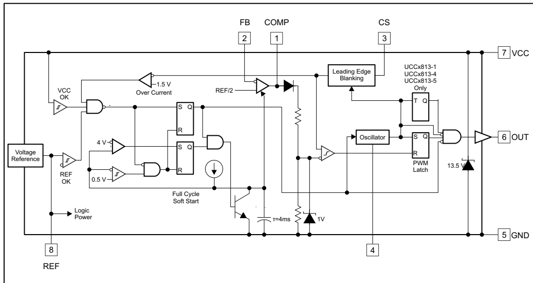
方框图
