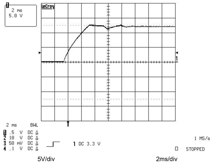
图 8-10. 满载启动条件下的输出电压行为
