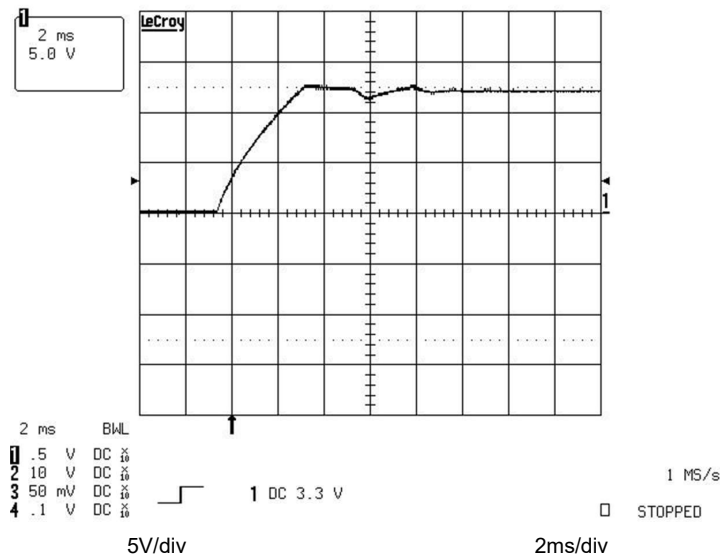
图 8-10. 满载启动条件下的输出电压行为
