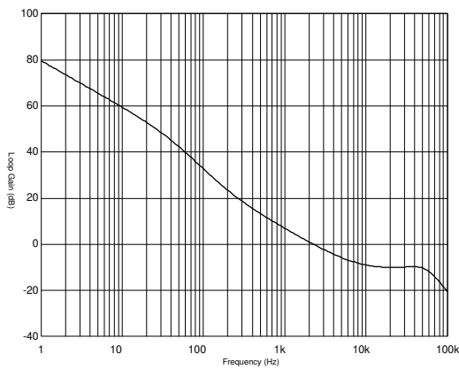
图 8-4. 转换器闭环波特图：增益
