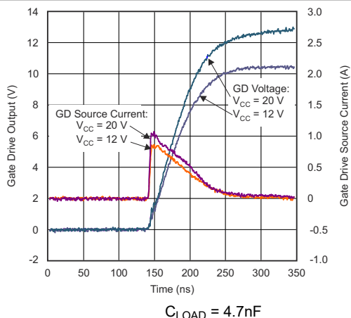
图 6-13. 栅极驱动上升与时间间的关系
