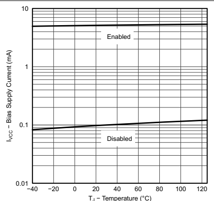
图 6-2. 辅助电源电流与温度间的关系
