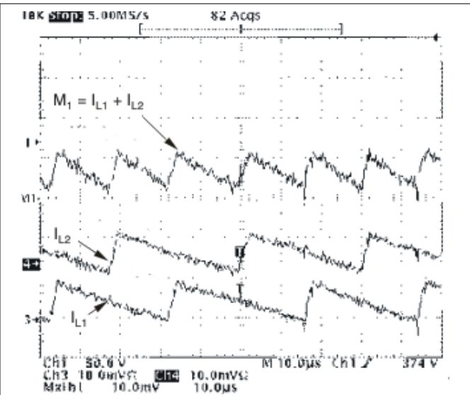
图 8-3. 265V RMS 输入时峰值线路电压条件下的电感器和输入纹波电流
