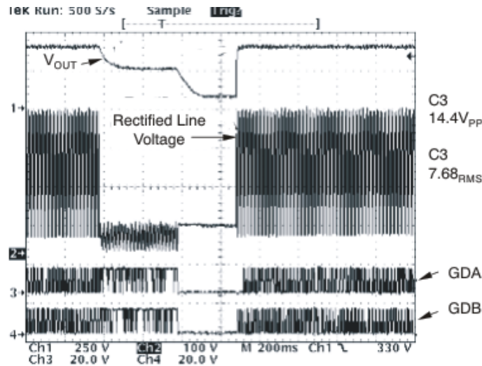
图 8-5. UCC28063A 在 265VRMS 下对线路欠压事件的响应
