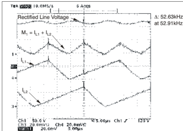
图 8-2. 85V RMS 时线路电压峰值条件下的电感器和输入纹波电流
