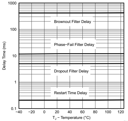
图 6-21. 各种延迟时间与温度间的关系
