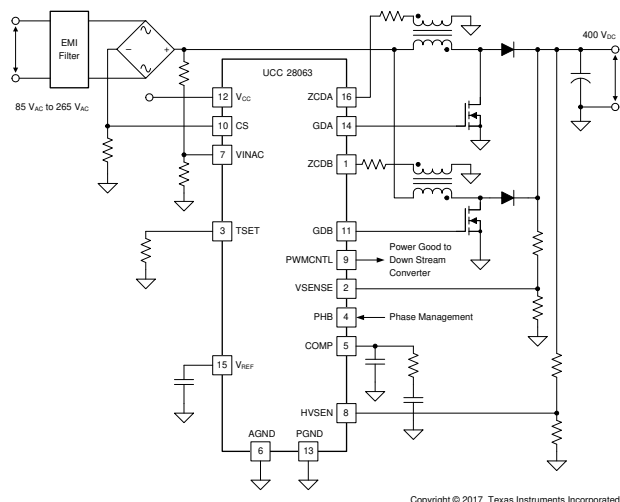
典型应用图
