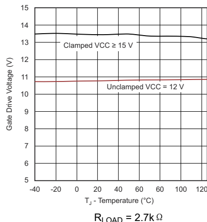
图 6-18. 栅极驱动高电压与温度间的关系
