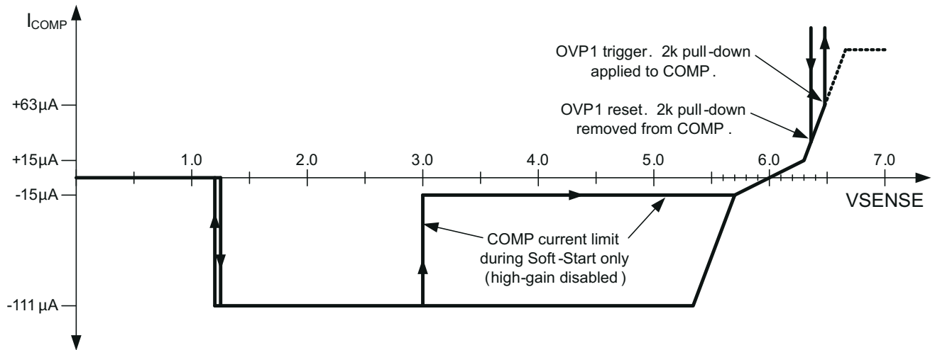
图 7-5. 扩展的 COMP 输出电流曲线
