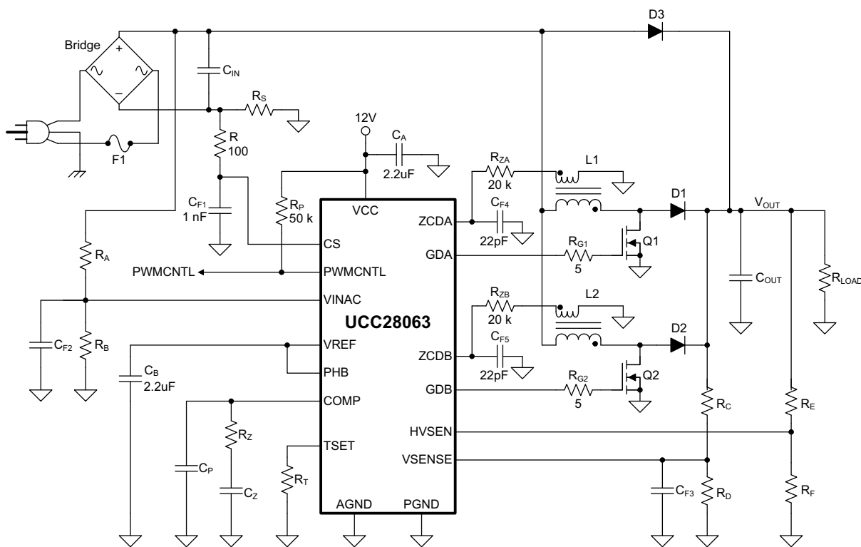
图 8-1. 典型交错转换模式 PFC 前置稳压器
