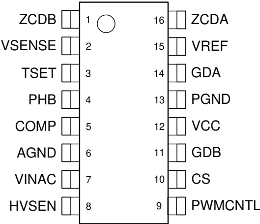
图 5-1. D 封装 16 引脚 SOIC 顶视图
