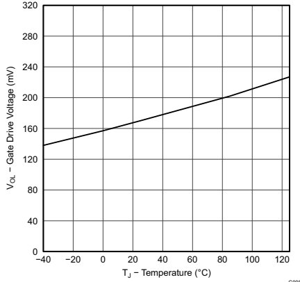
图 6-19. 栅极驱动低电压与温度间的关系
