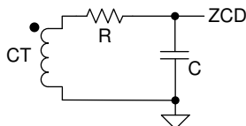
图 7-1. 简单的 RC 延迟电路
