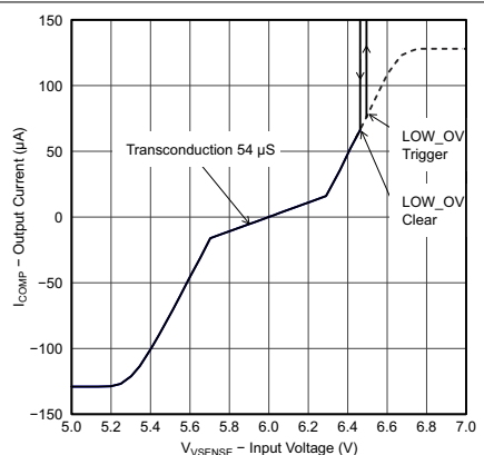
图 6-5. 误差放大器输出电流与输入电压间的关系
