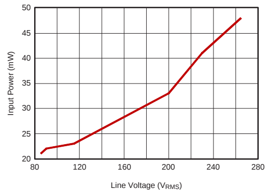
待机功耗
