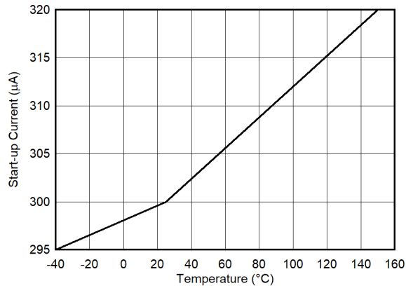
图 5-3. 启动电流和静态电流
