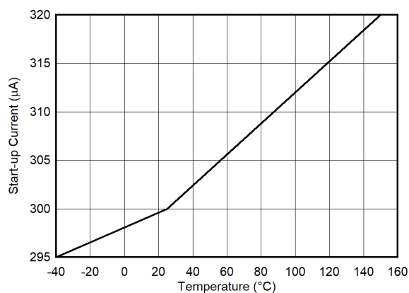
图 5-3. 启动电流和静态电流
