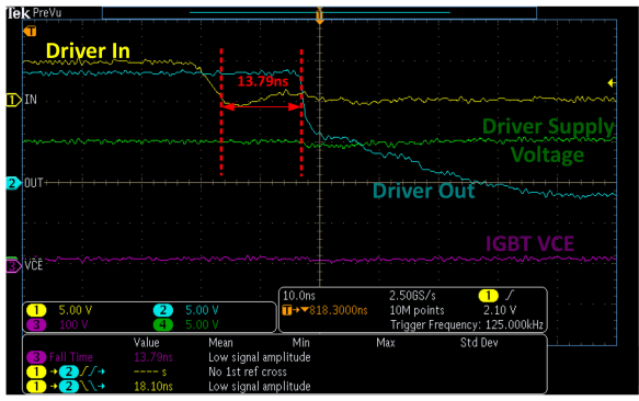
图 7-5. 关断传播延迟波形
