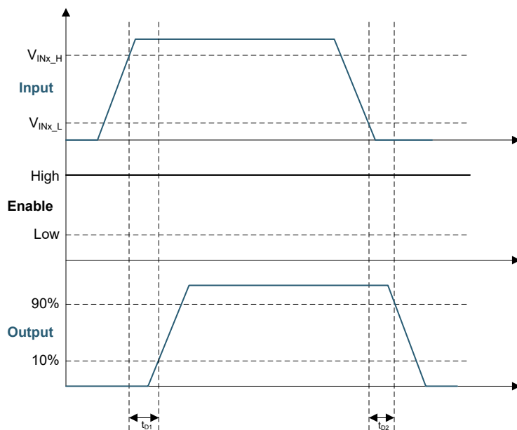
图 5-2. 输入/输出运行
