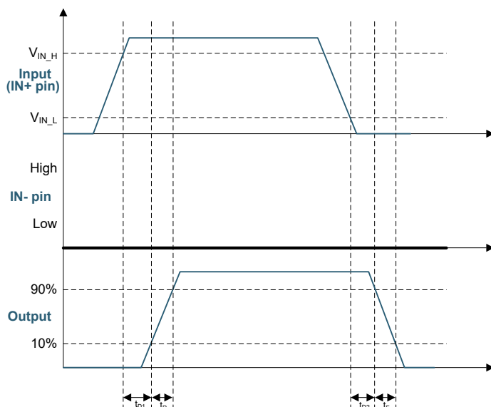
图 5-2. 双输入版本， IN+ = \text{PWM} ， IN- = \text{GND}
