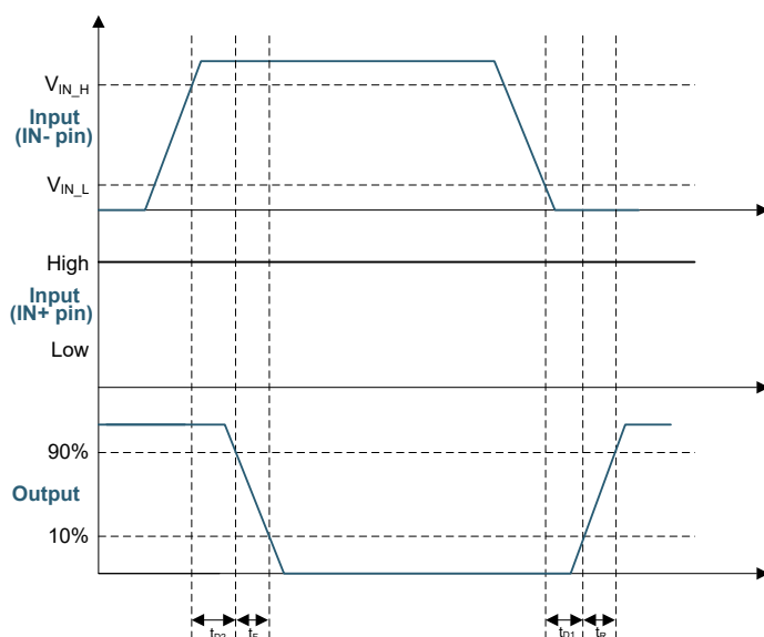
图 5-3. 双输入版本， IN- = \text{PWM} ， IN+ = \text{高电平 (或 VDD)}
