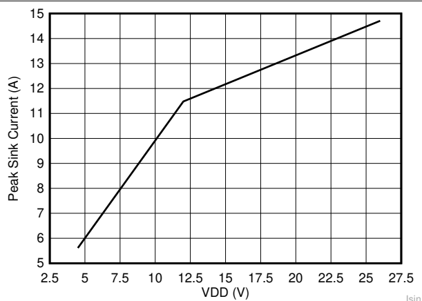
图 5-5. 峰值灌电流与 V_{DD} 间的关系
