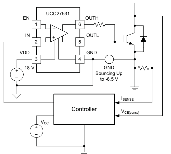
无需负偏压即可驱动 IGBT
