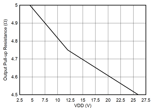
图 6-12. 输出上拉电阻
