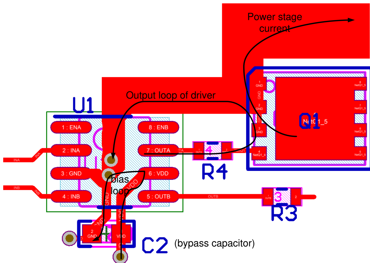
图 10-1. UCC27524A-Q1 布局示例
