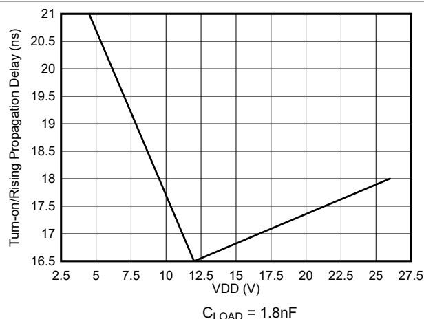
图 6-17. 输入到输出上升 (导通) 传播延迟与 VDD 间的关系
