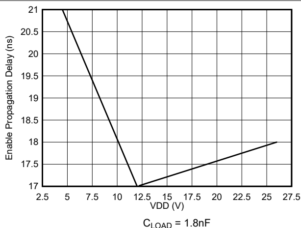
图 6-20. 使能到输出上升传播延迟
