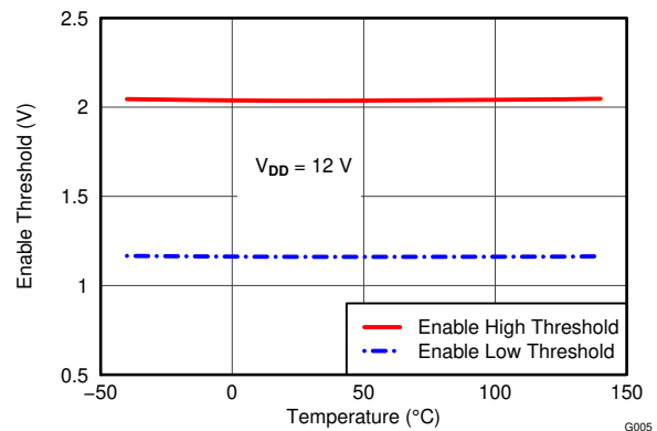
图 6-10. 启用阈值与温度间的关系
