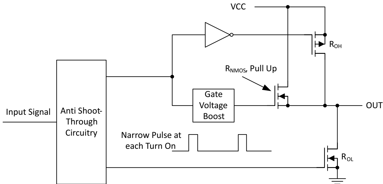
图 7-6. UCC2752x 栅极驱动器输出结构
