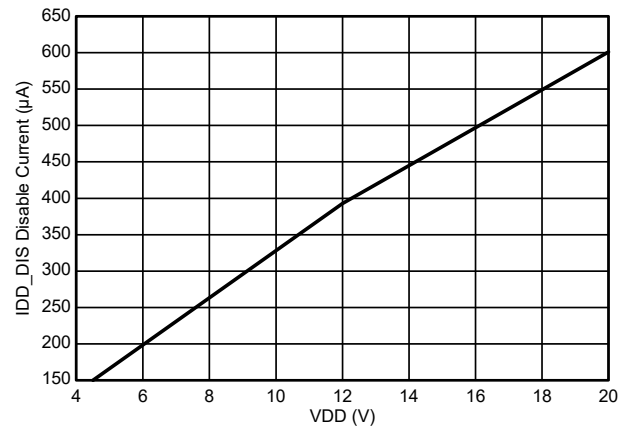
图 6-6. Disable Current (EN = 0 V)
