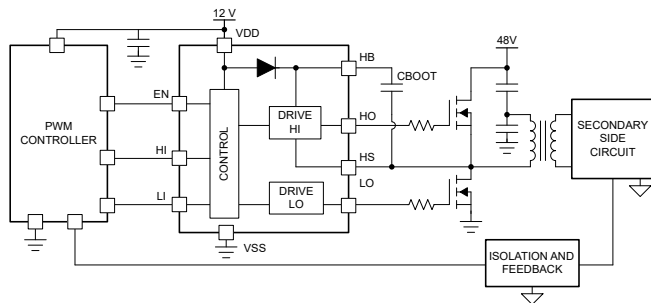
典型应用图
