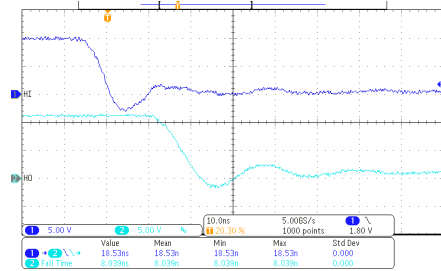
C_L = 1\text{nF} V_{DD} = 12\text{V} 图 7-5. HO 下降时间和 HI 至 HO 关断传播延迟
