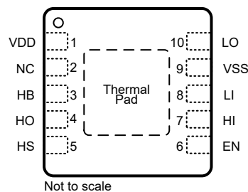
图 4-2. DRC 封装 10 引脚 SON 顶视图
