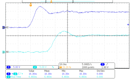
C_L = 1\text{nF} V_{DD} = 12\text{V} 图 7-4. HO 上升时间和 HI 至 HO 导通传播延迟
