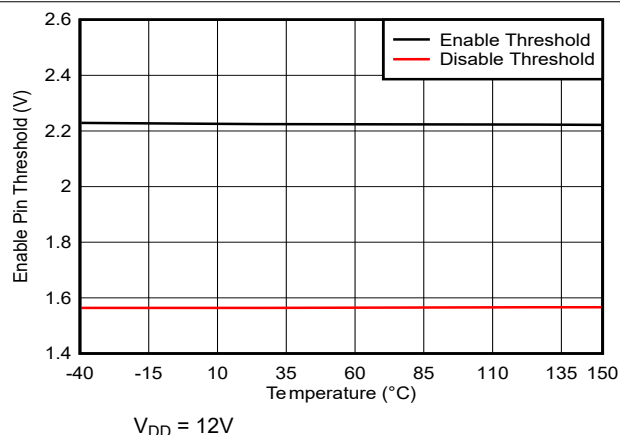
图 5-7. 启用阈值与温度间的关系
