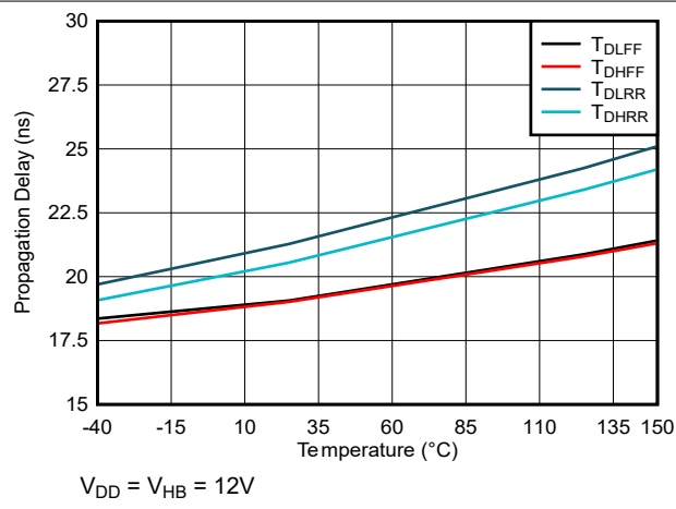
图 5-12. 传播延迟与温度间的关系
