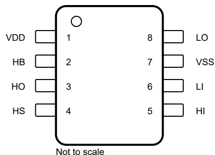
图 4-1. D 封装 8 引脚 SOIC 顶视图
