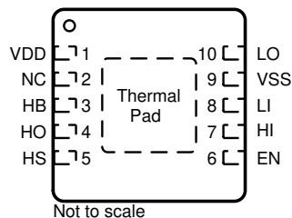
图 5-2. DRC 封装 10 引脚 SON 顶视图
