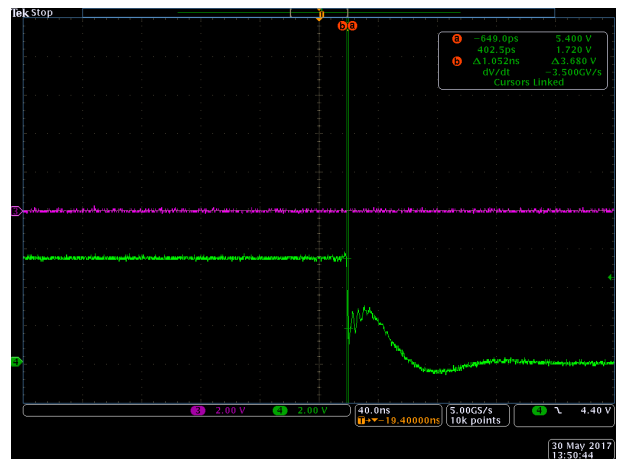
图 8-4. HO Fall Time
